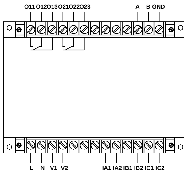
AMDGH-□/D202 系列保护器主单元接线端子图
