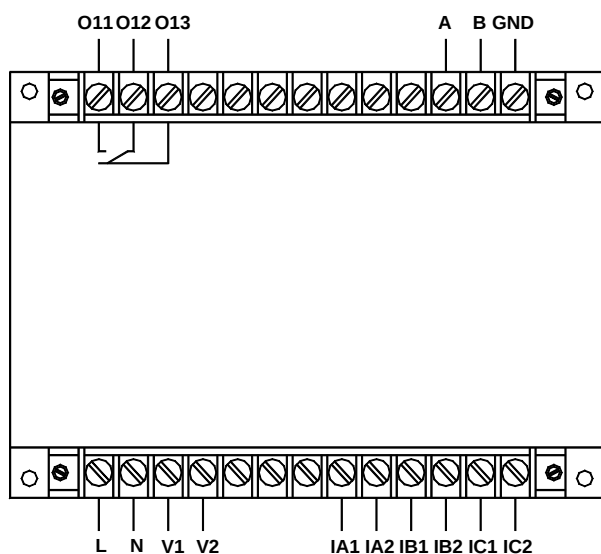
AMDGH-□/D201 系列保护器主单元接线端子图
