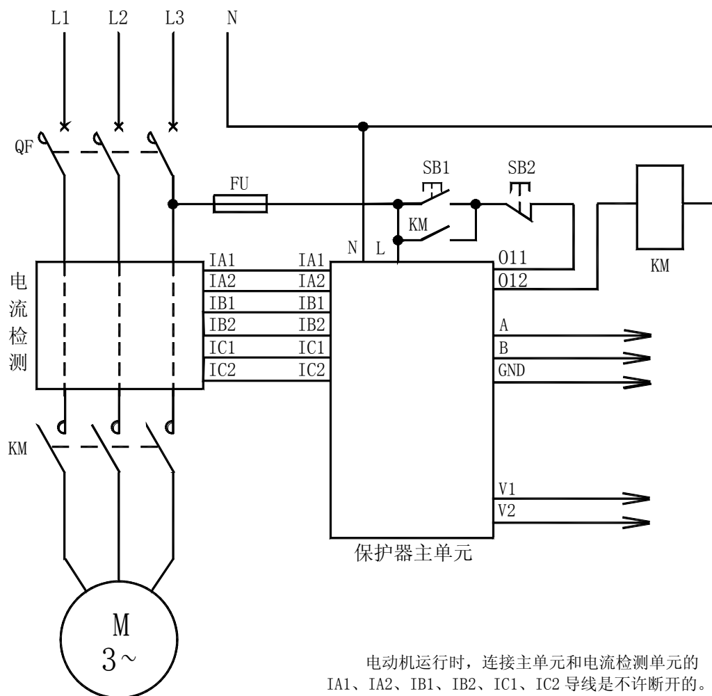
AMDGH-□/D20□ 系列电动机保护器应用电气原理图
