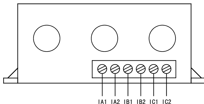
AMDGH-□/D20□ 系列保护器电流检测单元接线端子图
