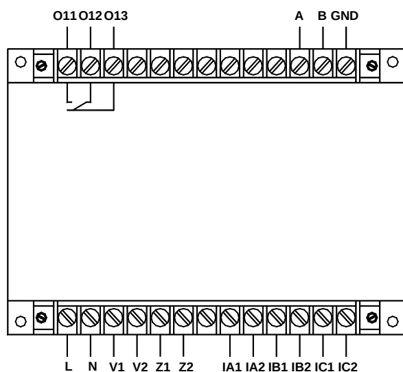
AMDGH-□/D211 系列保护器主单元接线端子图
