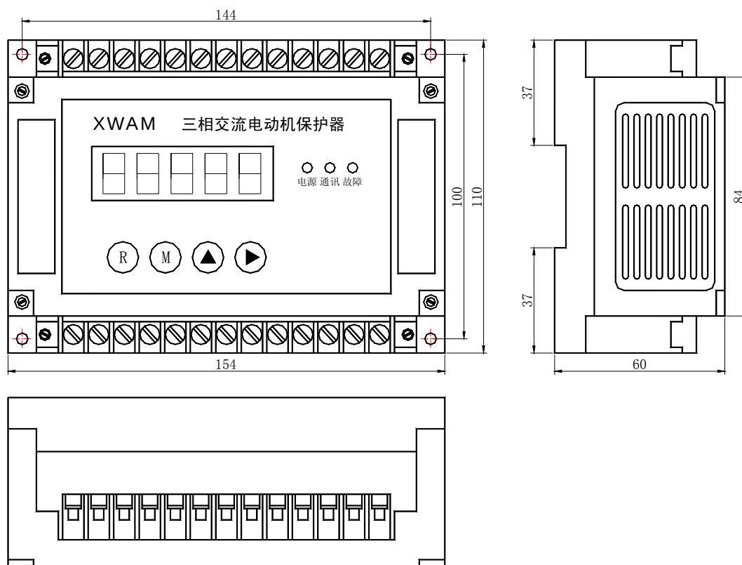
AMDGH-□/□/D21□ 系列电动机保护器主单元外形及安装孔尺寸
