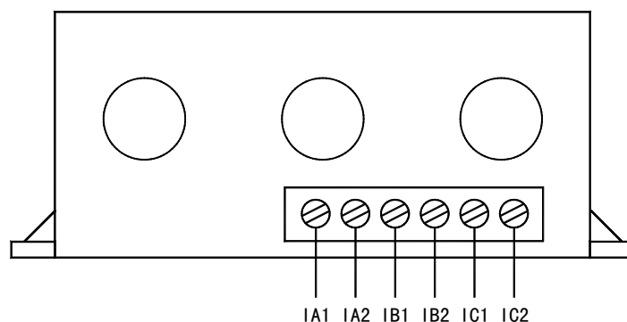
AMDGH-□/D21□ 系列保护器电流检测单元接线端子图
