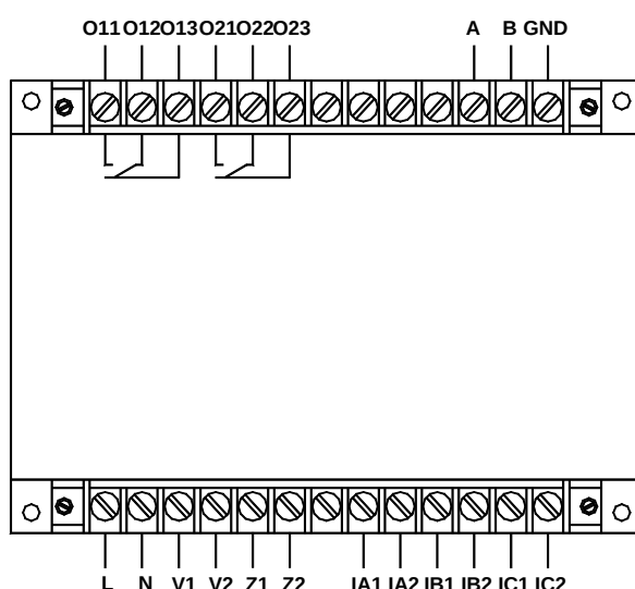
AMDGH-□/D212 系列保护器主单元接线端子图
