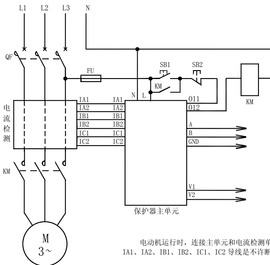
AMDGH-□/D22□ 系列电动机保护器应用电气原理图
