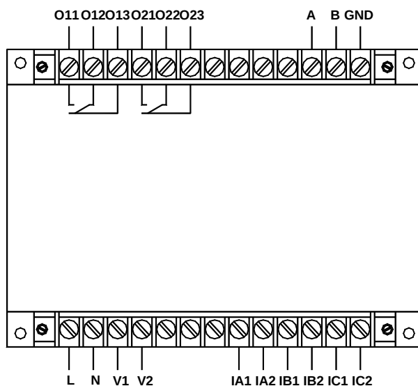
AMDGH-□/D222 系列保护器主单元接线端子图
