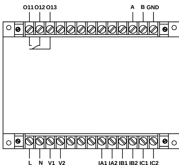
AMDGH-□/D221 系列保护器主单元接线端子图
