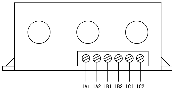
AMDGH-□/D22□ 系列保护器电流检测单元接线端子图
