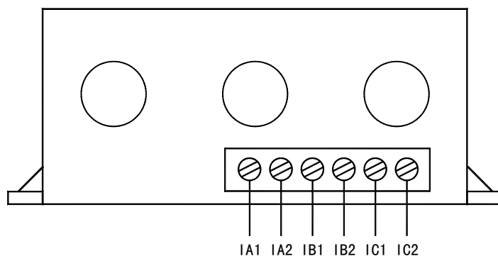
AMDGH-□/D23□ 系列保护器电流检测单元接线端子图
