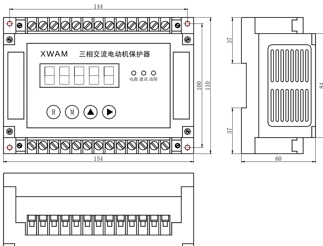
AMDGH-□/D23□ 系列电动机保护器主单元外形及安装孔尺寸
