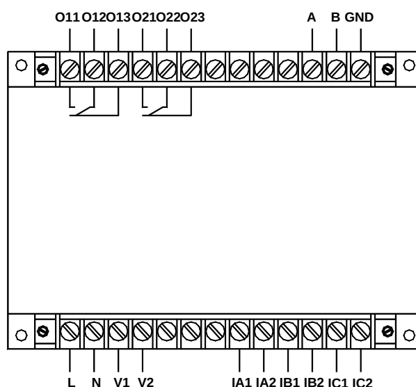
AMDGH-□/D232 系列保护器主单元接线端子图
