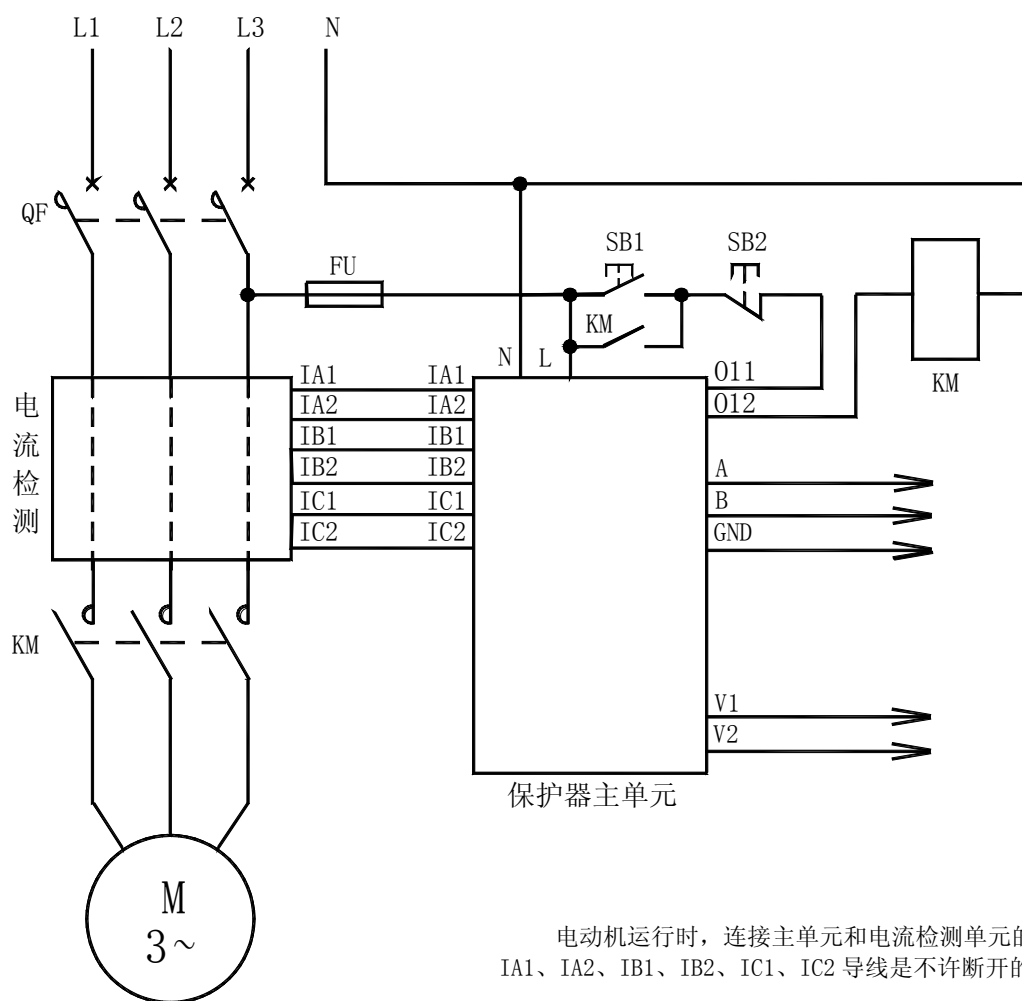
AMDGH-□/D23□ 系列电动机保护器应用电气原理图
