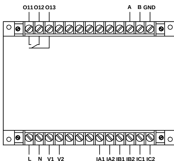
AMDGH-□/D231 系列保护器主单元接线端子图
