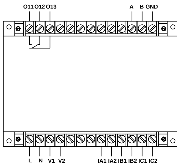
AMDGH-□/D241 系列保护器主单元接线端子图
