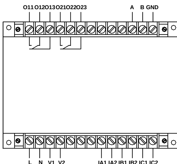
AMDGH-□/D242 系列保护器主单元接线端子图
