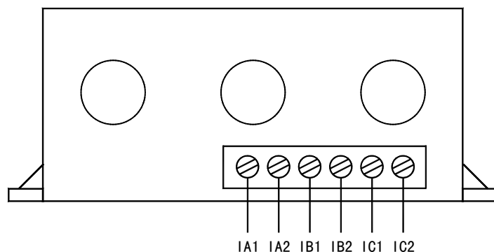
AMDGH-□/D24□ 系列保护器电流检测单元接线端子图
