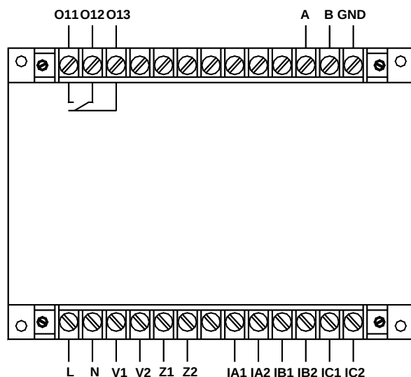
AMDGH-□/D251 系列保护器主单元接线端子图
