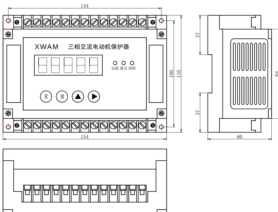
AMDGH-□/D25□ 系列电动机保护器主单元外形及安装孔尺寸
