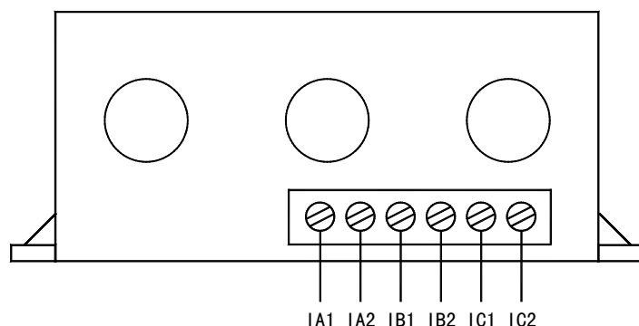
AMDGH-□/D25□ 系列保护器电流检测单元接线端子图
