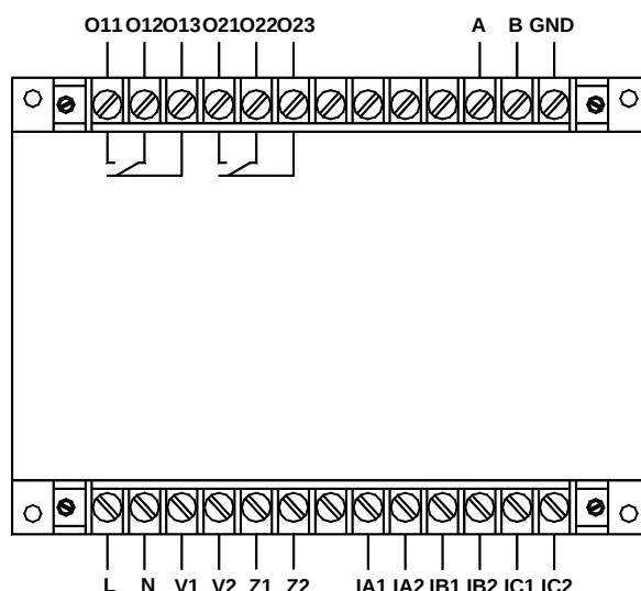
AMDGH-□/D252 系列保护器主单元接线端子图
