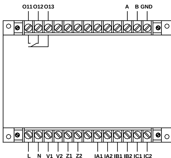
AMDGH-□/D261 系列保护器主单元接线端子图
