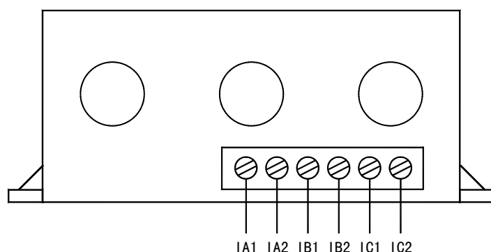
AMDGH-□/D26□ 系列保护器电流检测单元接线端子图
