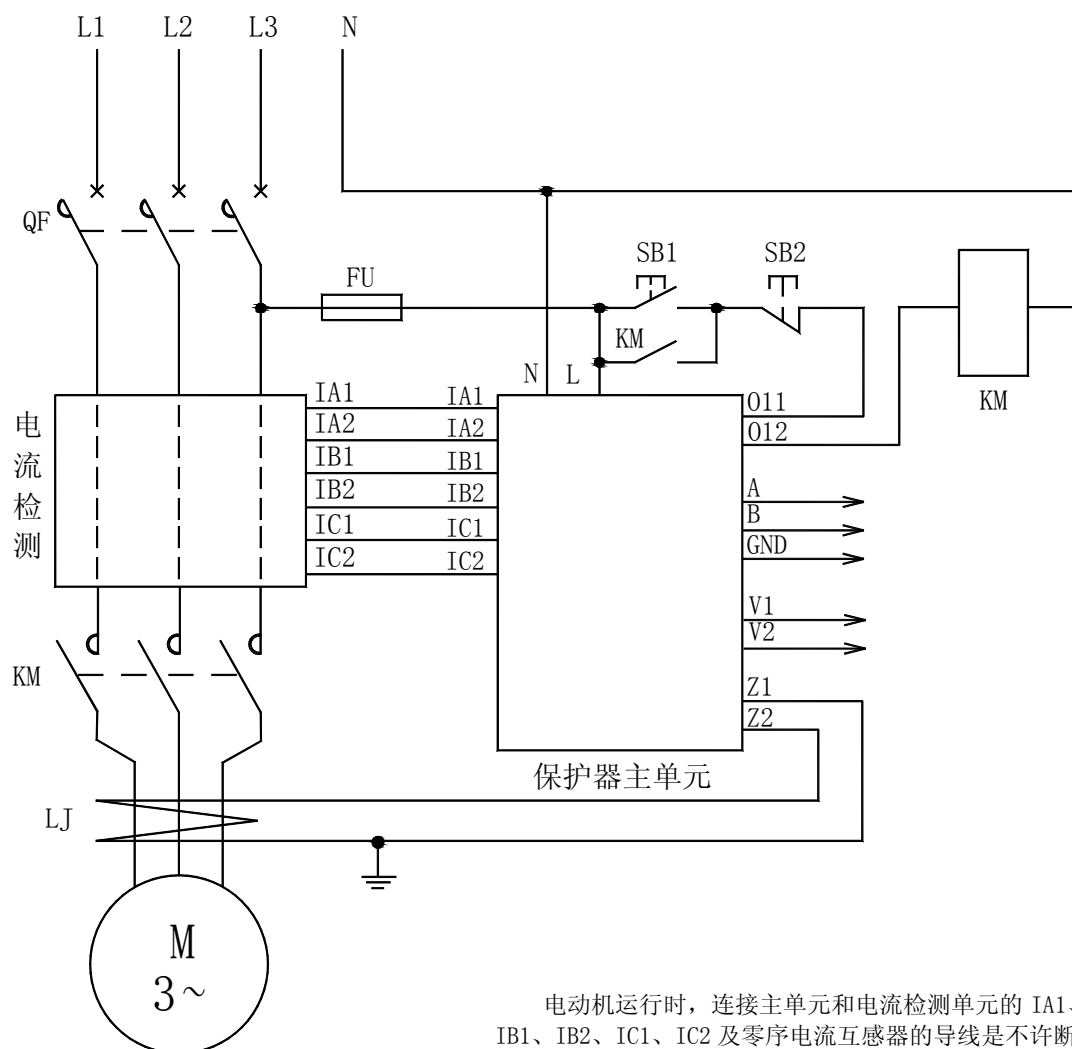
AMDGH-□/D26□ 系列电动机保护器应用电气原理图
