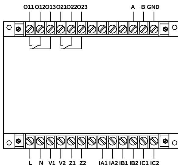
AMDGH-□/D262 系列保护器主单元接线端子图
