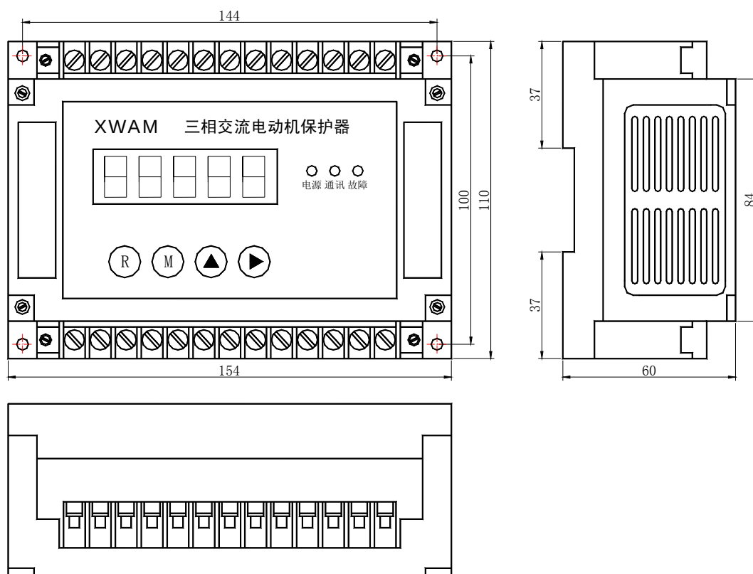
AMDGH-□/D26□ 系列电动机保护器主单元外形及安装孔尺寸
