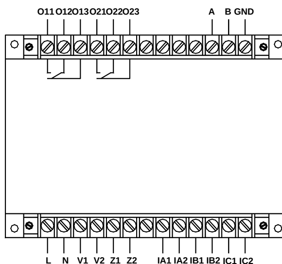
AMDGH-□/D272 系列保护器主单元接线端子图
