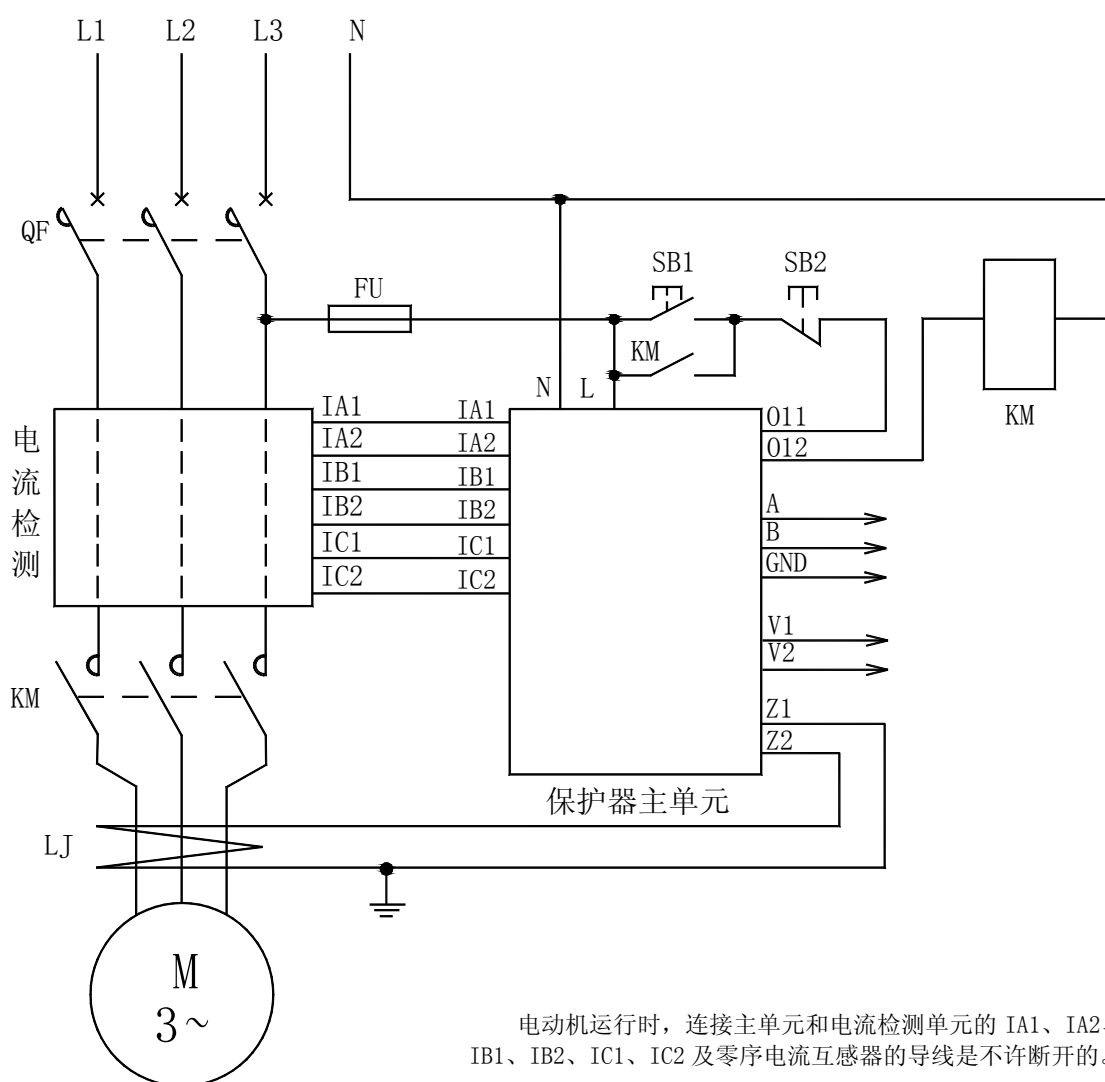
AMDGH-□/D27□ 系列电动机保护器应用电气原理图
