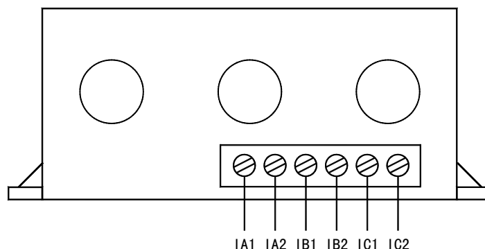
AMDGH-□/D27□ 系列保护器电流检测单元接线端子图
