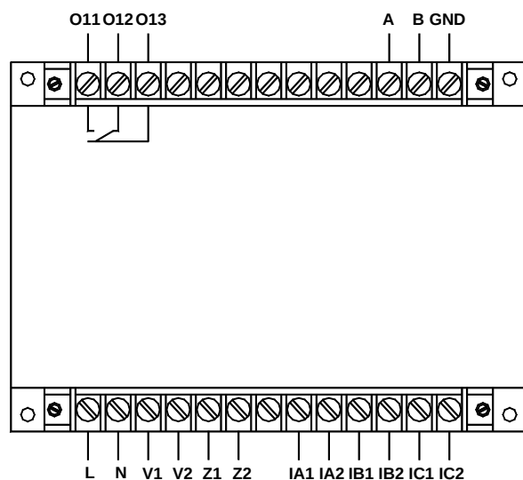
AMDGH-□/D271 系列保护器主单元接线端子图
