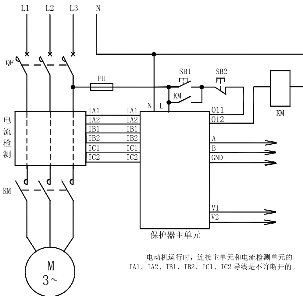
AMDGH-□/D30□ 系列电动机保护器应用电气原理图
