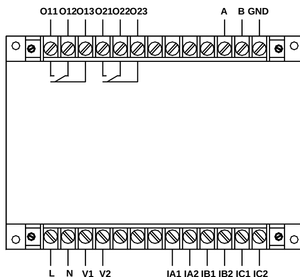
AMDGH-□/D302 系列保护器主单元接线端子图
