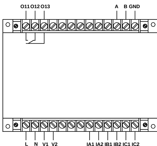
AMDGH-□/D301 系列保护器主单元接线端子图
