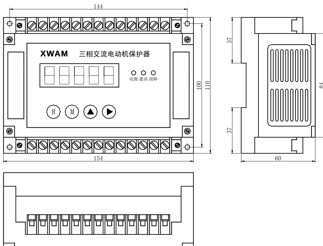
AMDGH-□/D30□ 系列电动机保护器主单元外形及安装孔尺寸
