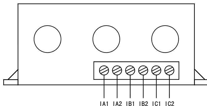
AMDGH-□/D30□ 系列保护器电流检测单元接线端子图
