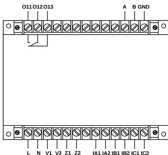
AMDGH-□/D311 系列保护器主单元接线端子图
