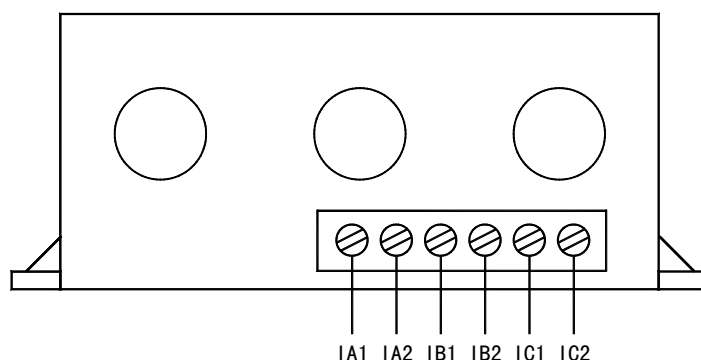
AMDGH-□/D31□ 系列保护器电流检测单元接线端子图
