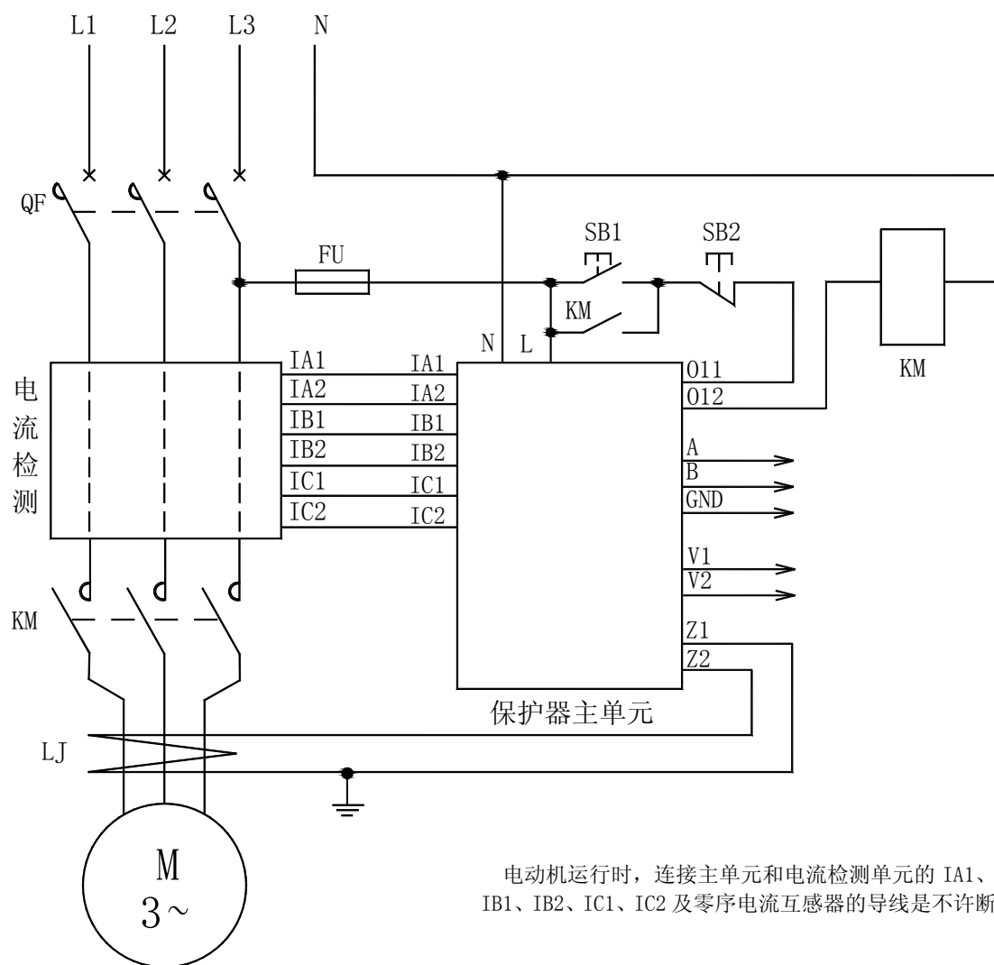
AMDGH-□/D31□ 系列电动机保护器应用电气原理图
