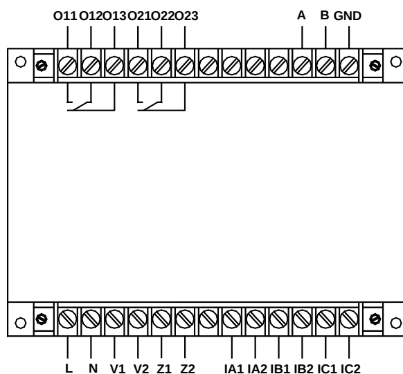
AMDGH-□/D312 系列保护器主单元接线端子图
