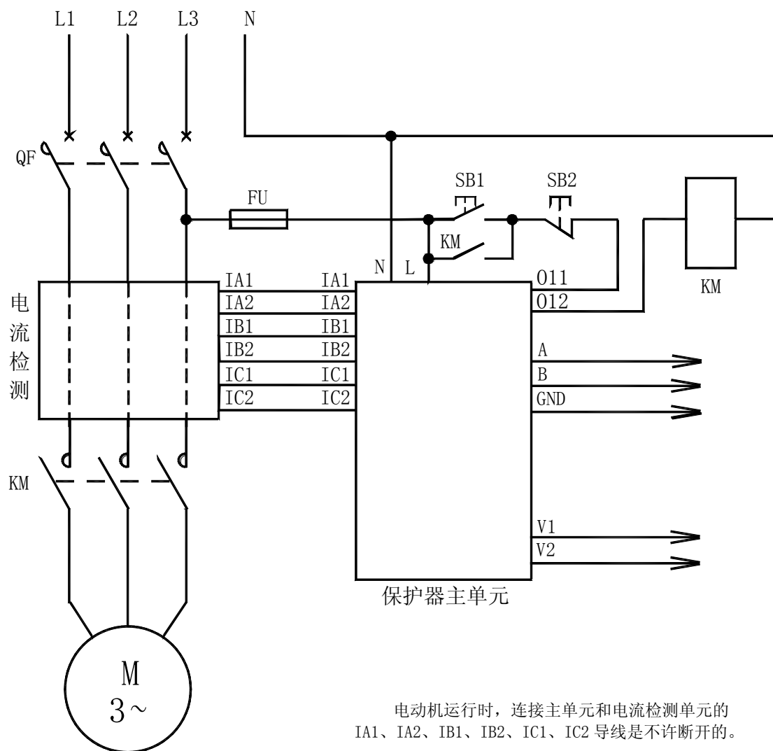
AMDGH-□/D33□ 系列电动机保护器应用电气原理图
