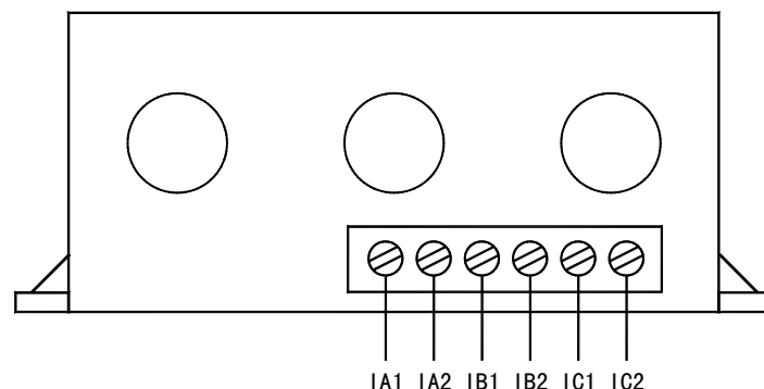
AMDGH-□/D33□ 系列保护器电流检测单元接线端子图
