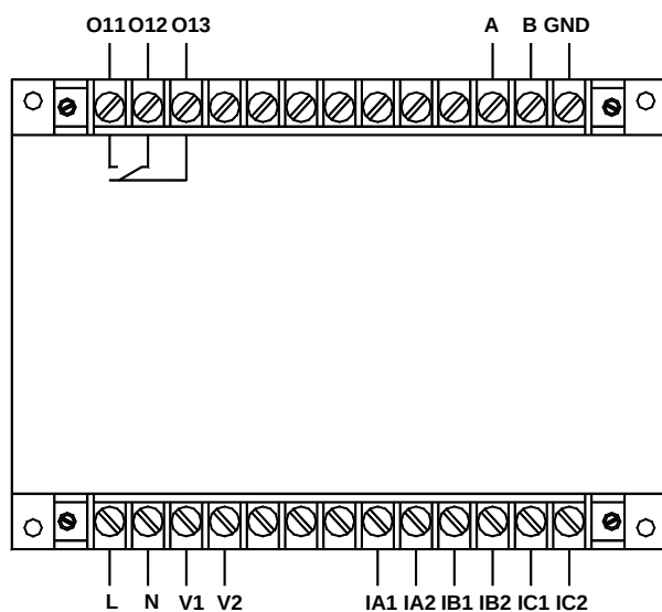
AMDGH-□/D331 系列保护器主单元接线端子图
