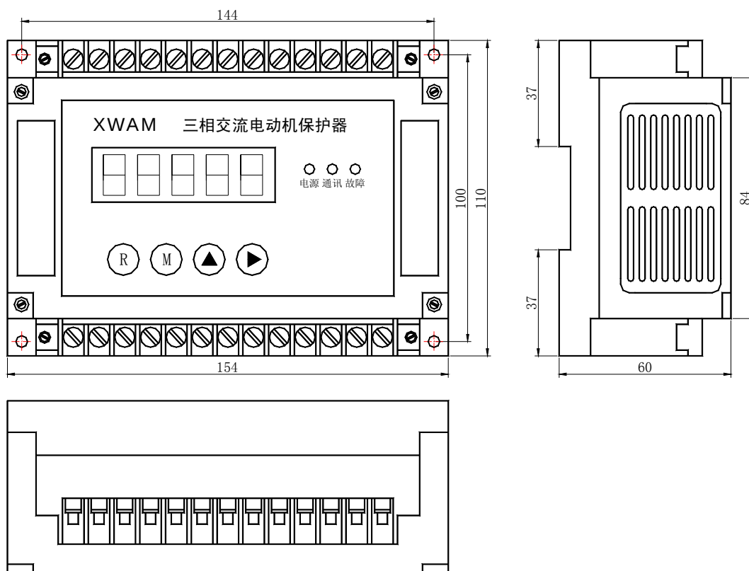
AMDGH-□/D33□ 系列电动机保护器主单元外形及安装孔尺寸
