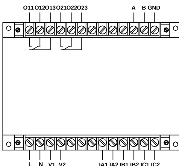
AMDGH-□/D332 系列保护器主单元接线端子图
