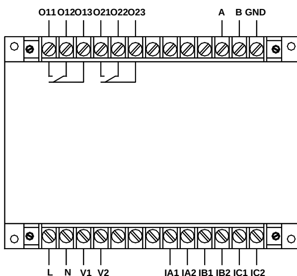
AMDGH-□/D342 系列保护器主单元接线端子图
