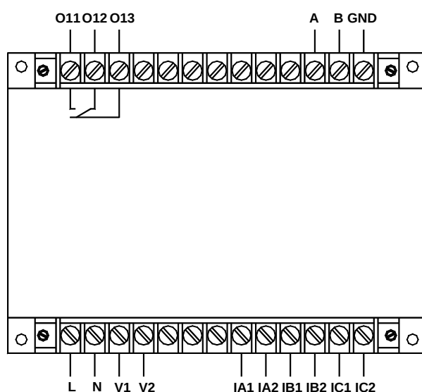
AMDGH-□/D341 系列保护器主单元接线端子图
