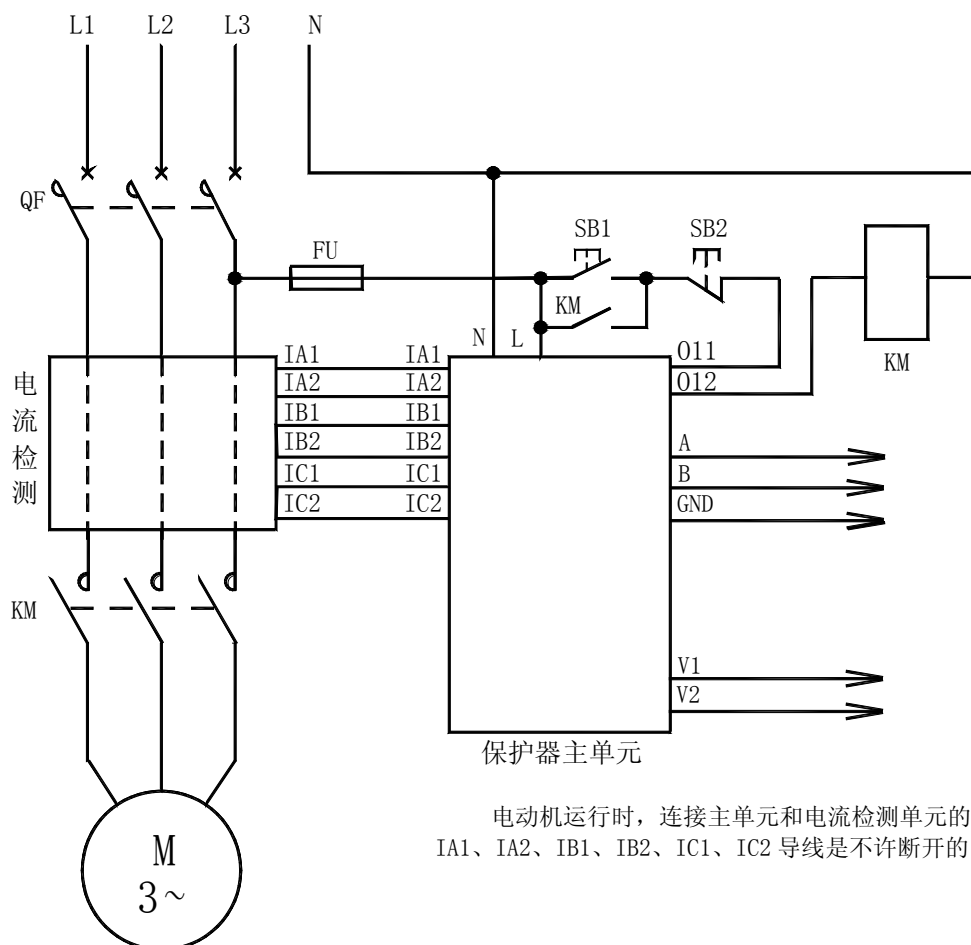
AMDGH-□/D34□ 系列电动机保护器应用电气原理图
