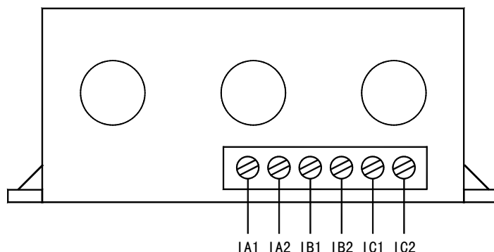
AMDGH-□/D34□ 系列保护器电流检测单元接线端子图
