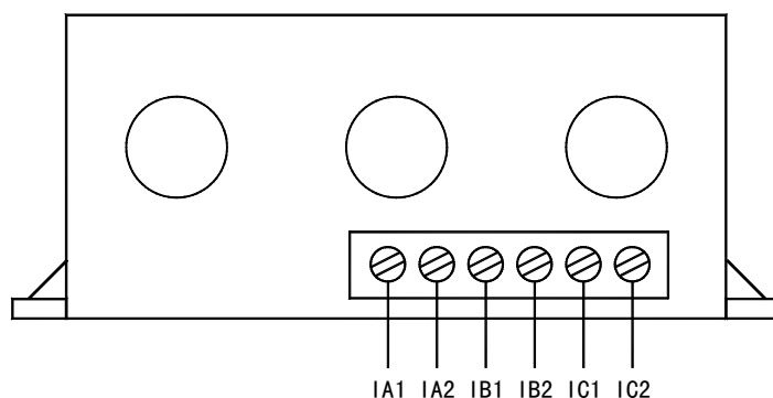
AMDGH-□/D35□ 系列保护器电流检测单元接线端子图
