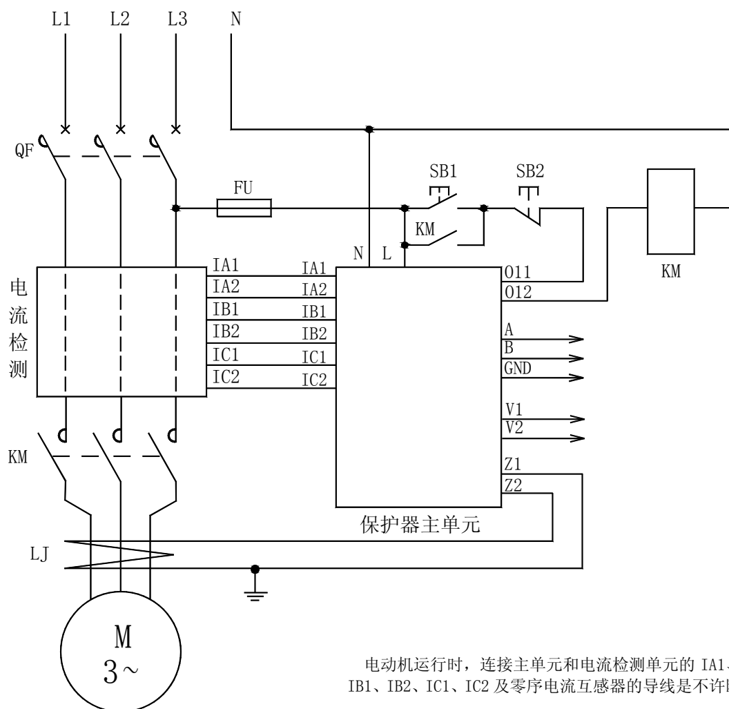
AMDGH-□/D35□ 系列电动机保护器应用电气原理图
