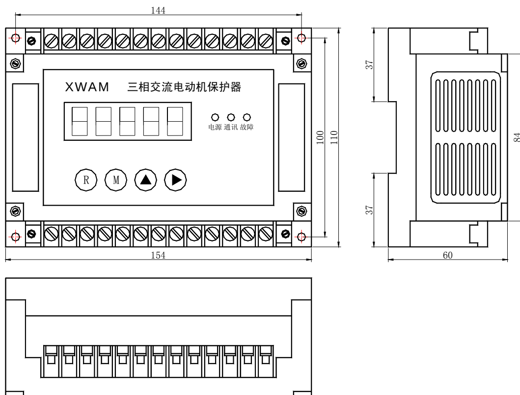
AMDGH-□/□D35□ 系列电动机保护器主单元外形及安装孔尺寸
