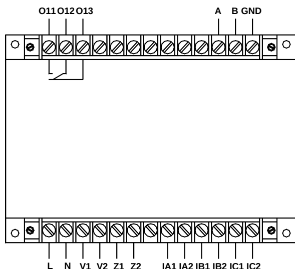
AMDGH-□/D351 系列保护器主单元接线端子图
