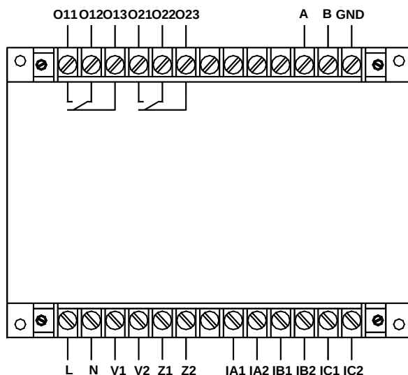
AMDGH-□/D352 系列保护器主单元接线端子图
