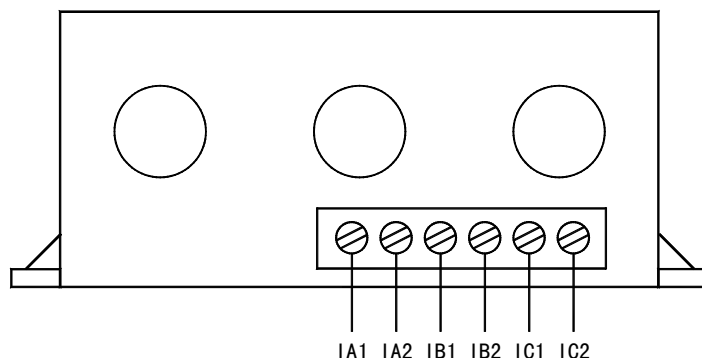
AMDGH-□/D36□ 系列保护器电流检测单元接线端子图
