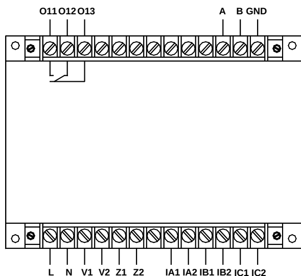
AMDGH-□/D361 系列保护器主单元接线端子图
