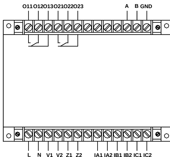
AMDGH-□/D362 系列保护器主单元接线端子图
