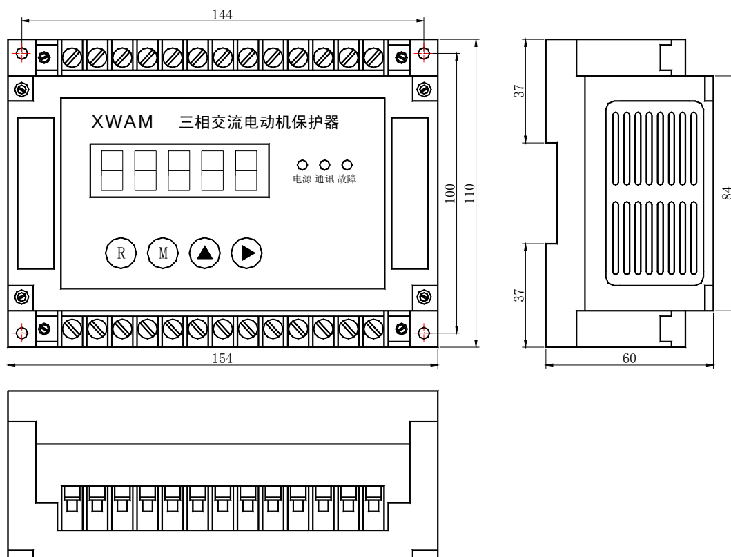
AMDGH-□/D36□ 系列电动机保护器主单元外形及安装孔尺寸
