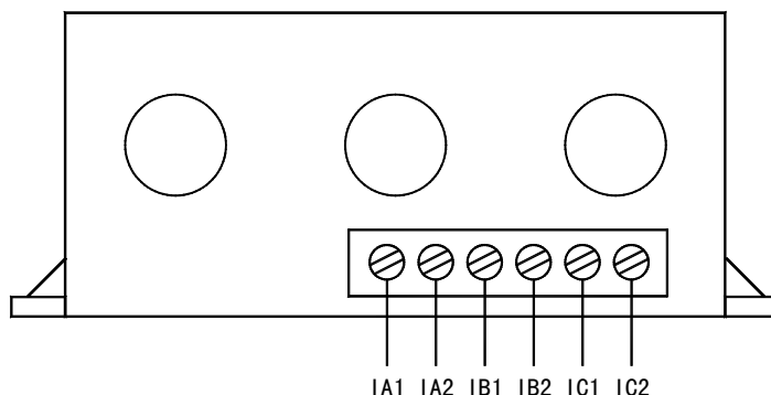
AMDGH-□/D37□ 系列保护器电流检测单元接线端子图
