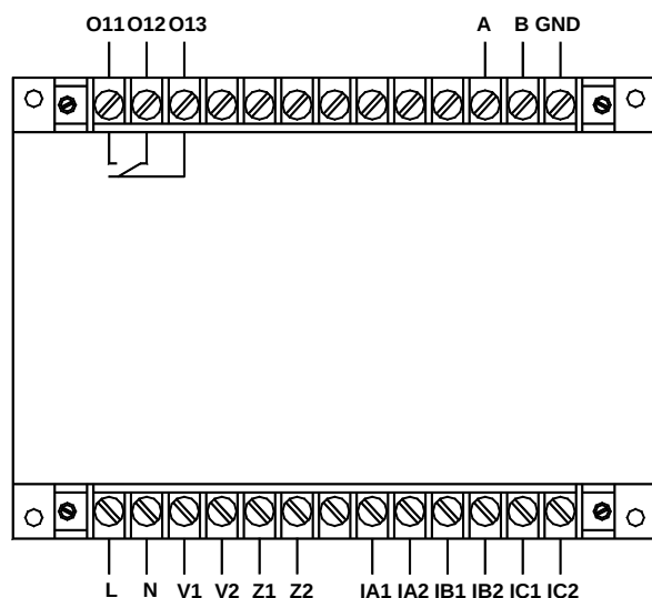
AMDGH-□/D371 系列保护器主单元接线端子图
