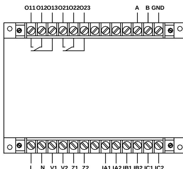
AMDGH-□/D372 系列保护器主单元接线端子图
