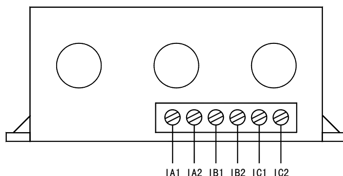
AMDGH-□/D40□ 系列保护器电流检测单元接线端子图
