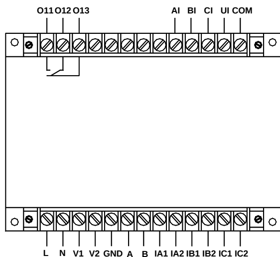
AMDGH-□/D401 系列保护器主单元接线端子图
