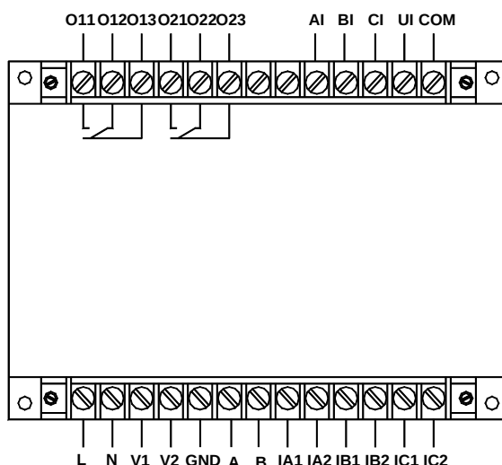
AMDGH-□/D402 系列保护器主单元接线端子图
