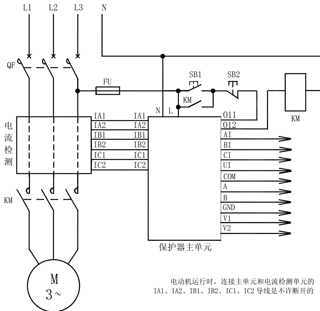
AMDGH-□/D40□ 系列电动机保护器应用电气原理图
