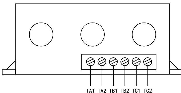
AMDGH-□/D42□ 系列保护器电流检测单元接线端子图
