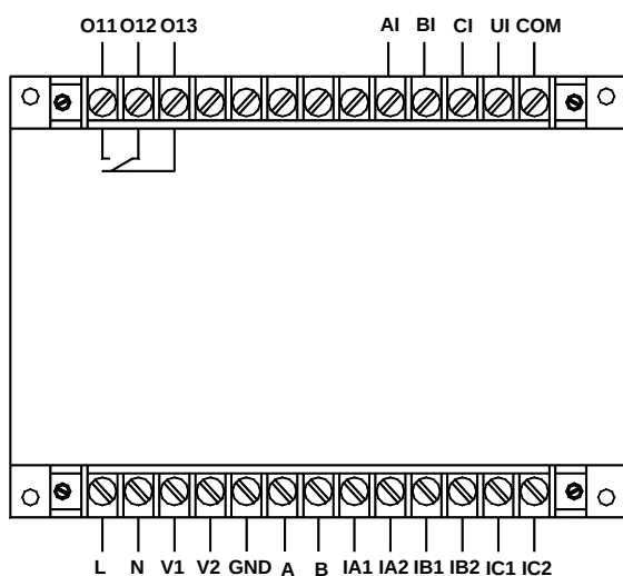
AMDGH-□/D421 系列保护器主单元接线端子图
