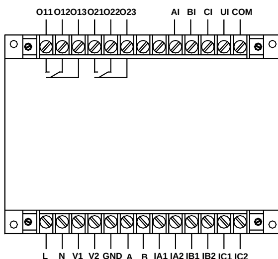
AMDGH-□/D422 系列保护器主单元接线端子图
