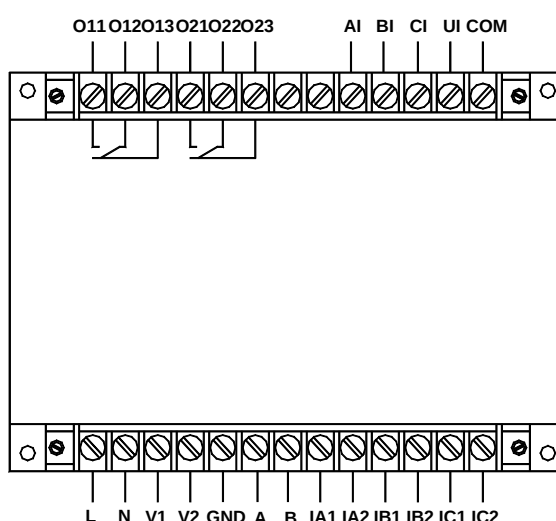
AMDGH-□/D432 系列保护器主单元接线端子图
