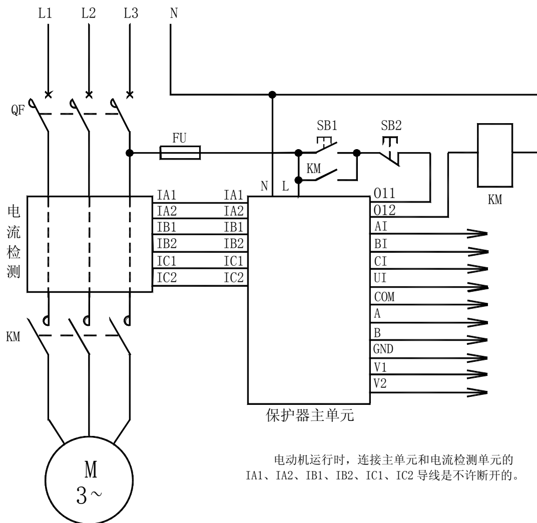
AMDGH-□/D43□ 系列电动机保护器应用电气原理图
