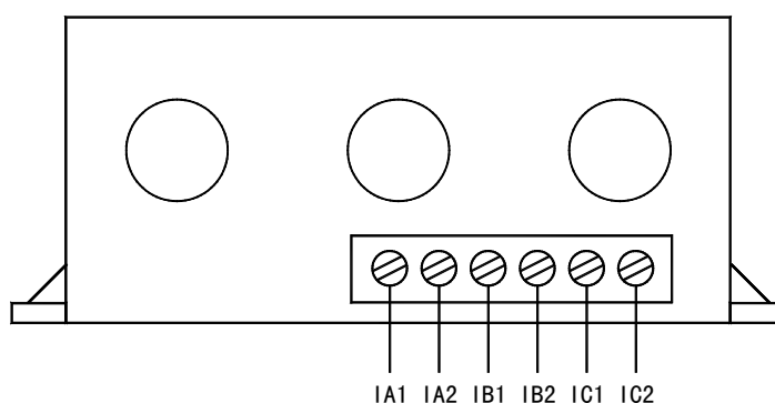
AMDGH-□/D43□ 系列保护器电流检测单元接线端子图
