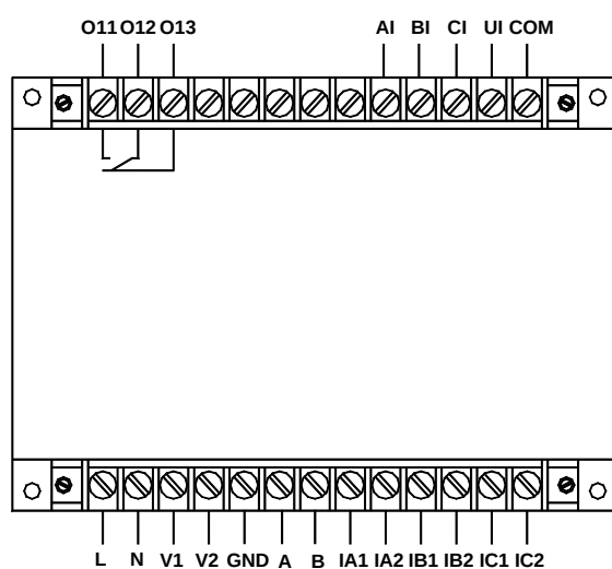
AMDGH-□/D431 系列保护器主单元接线端子图
