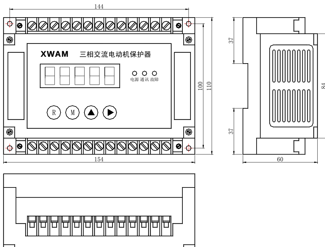
AMDGH-□/D43□ 系列电动机保护器主单元外形及安装孔尺寸
