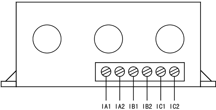
AMDGH-□/D44□ 系列保护器电流检测单元接线端子图
