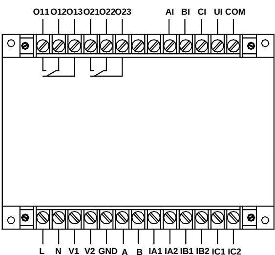
AMDGH-□/D442 系列保护器主单元接线端子图
