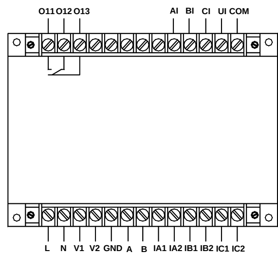
AMDGH-□/D441 系列保护器主单元接线端子图
