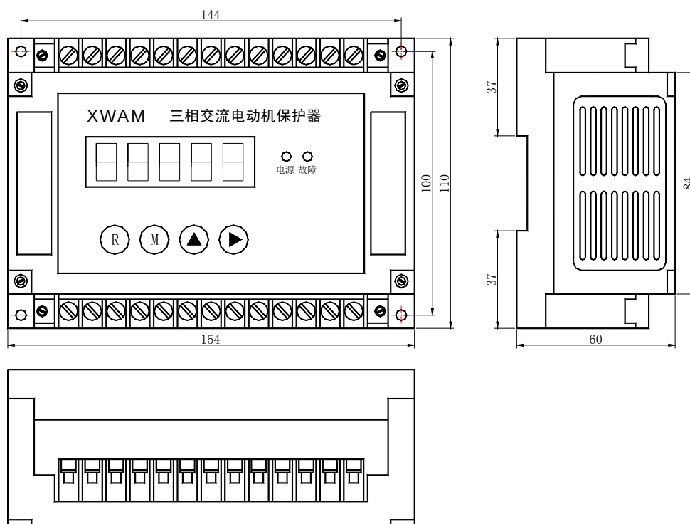
AMDGH-□/D521 系列电动机保护器主单元外形及安装尺寸
