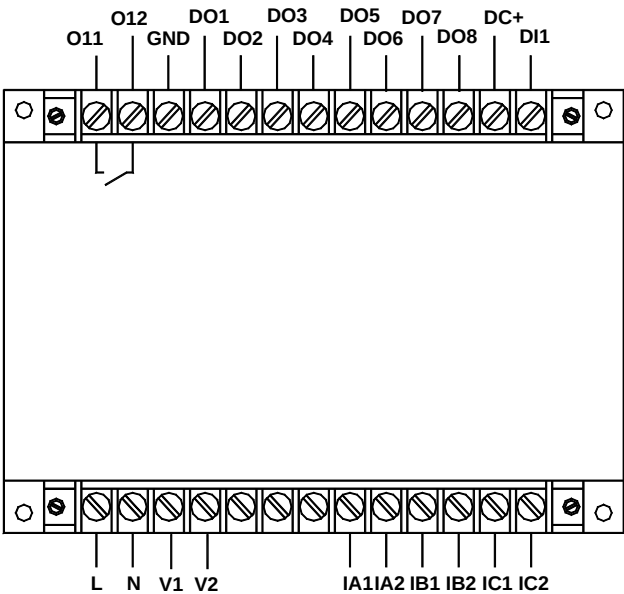
AMDGH-□/D521 系列保护器主单元接线端子图
