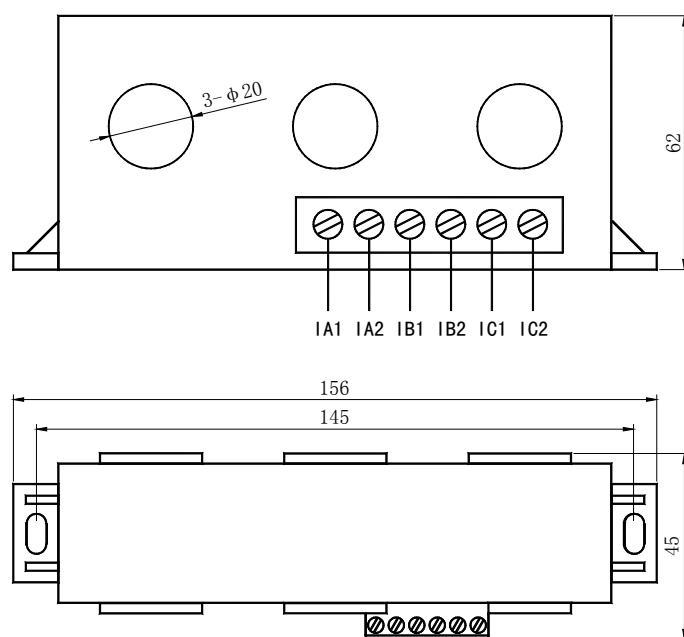
AMDGH-□/D521 系列电动机保护器电流检测单元外形及安装尺寸
