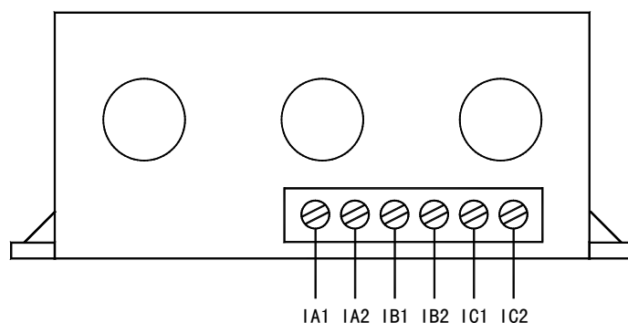
AMDGH-□/D521 系列保护器电流检测单元接线端子图
