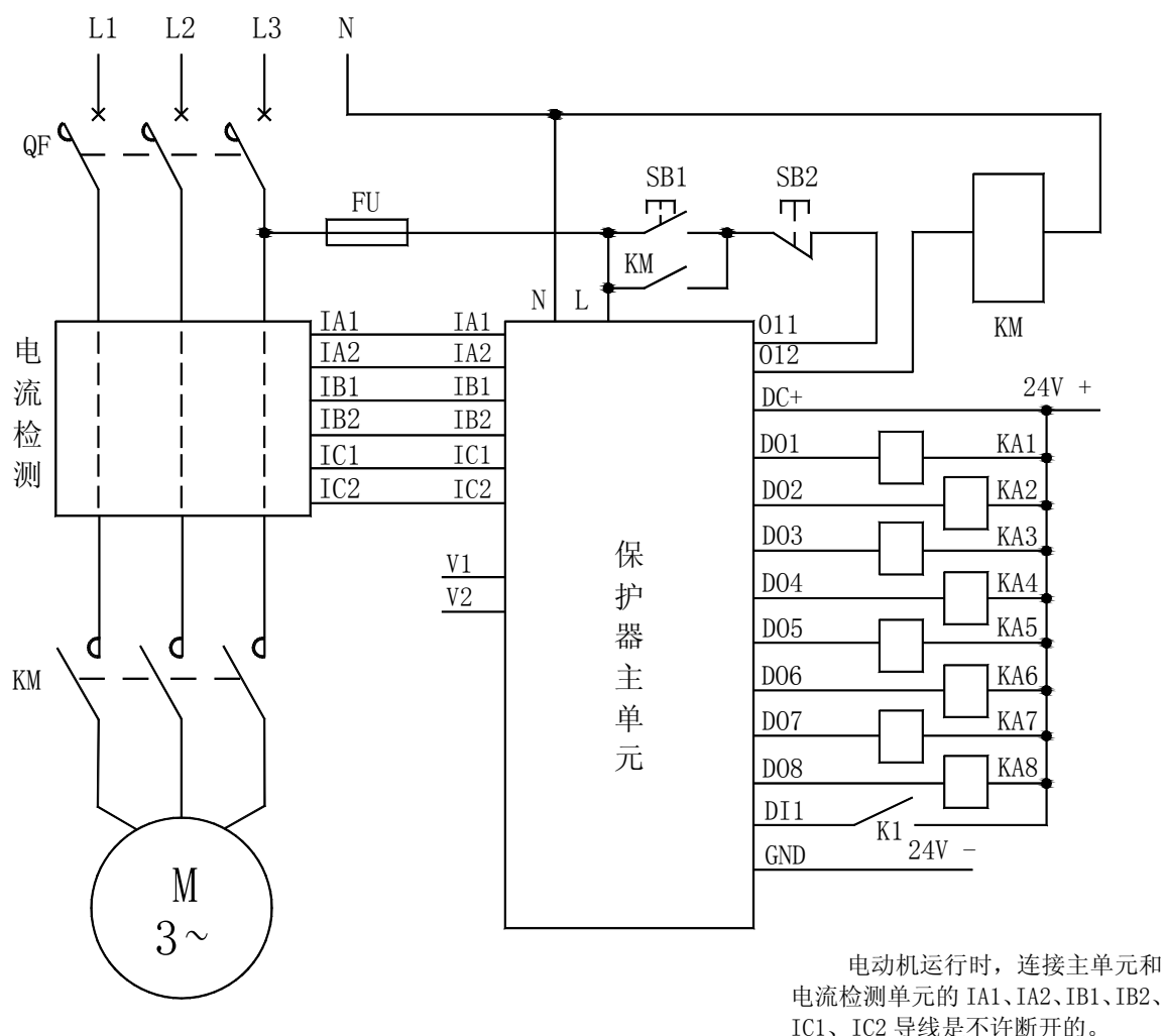
AMDGH-□/D521 系列电动机保护器 D0 连接继电器电气原理图
