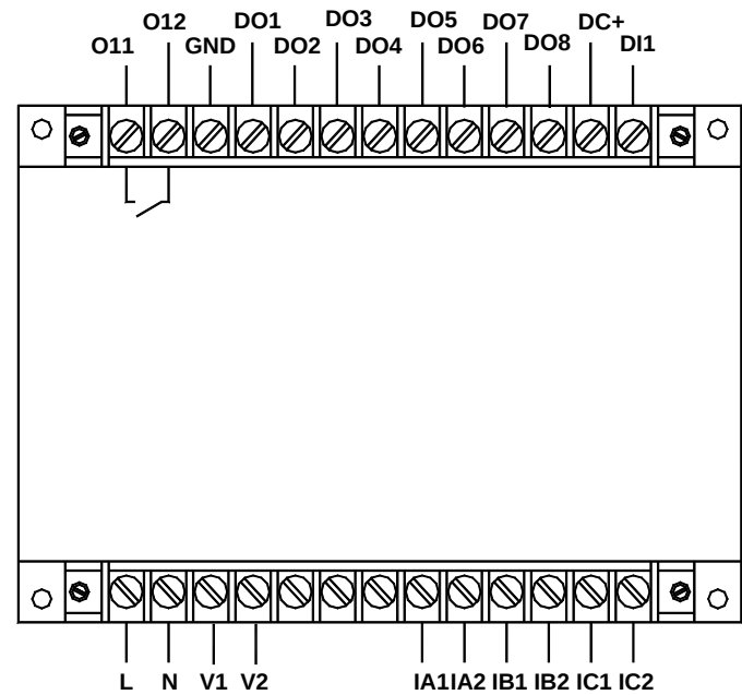
AMDGH-□/D531 系列保护器主单元接线端子图
