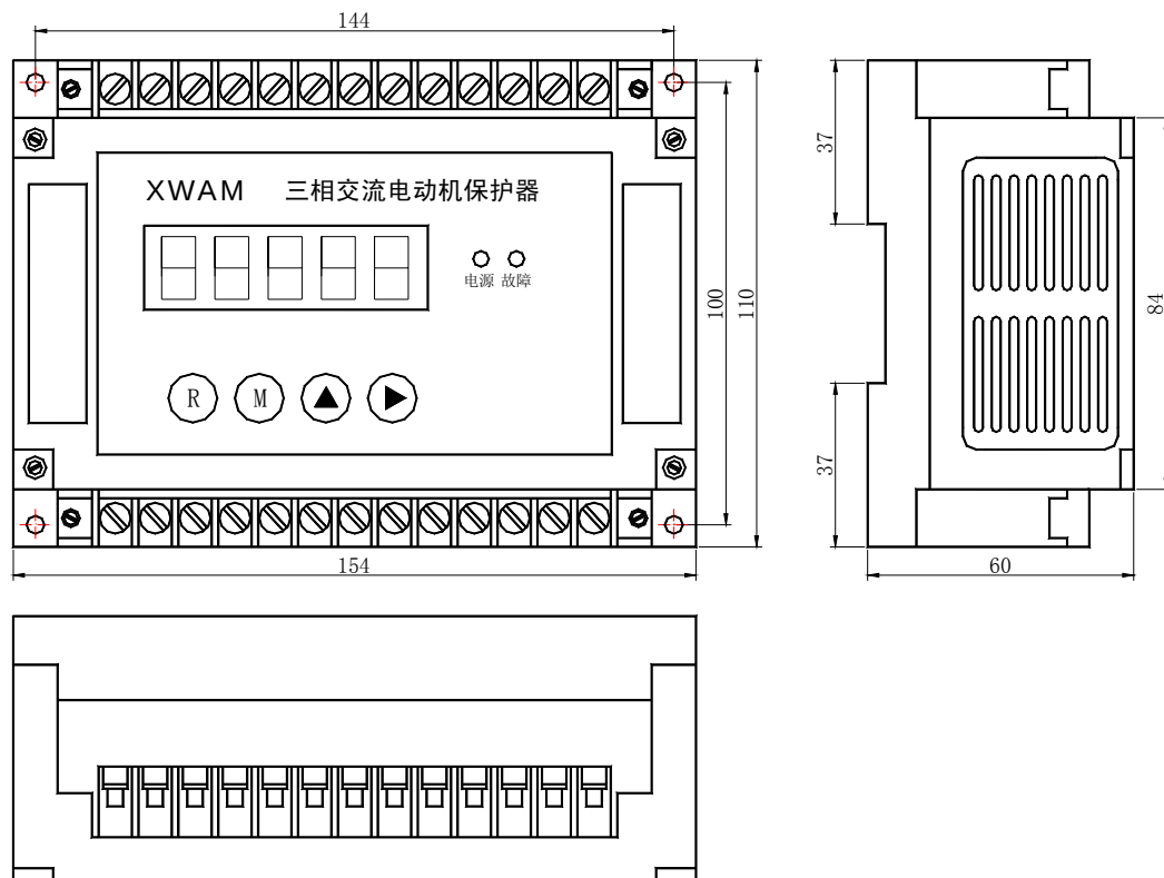
AMDGH-□/531 系列电动机保护器主单元外形及安装孔尺寸
