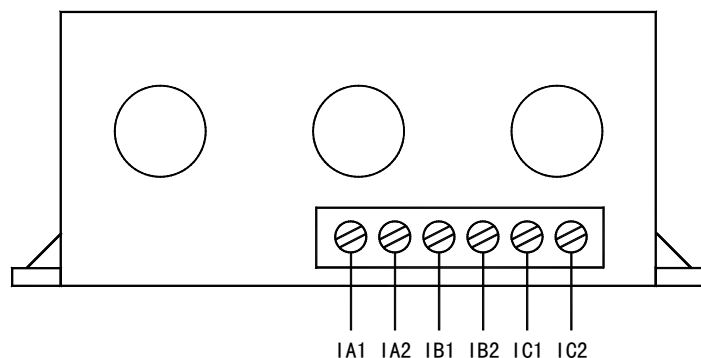
AMDGH-□/531 系列保护器电流检测单元接线端子图
