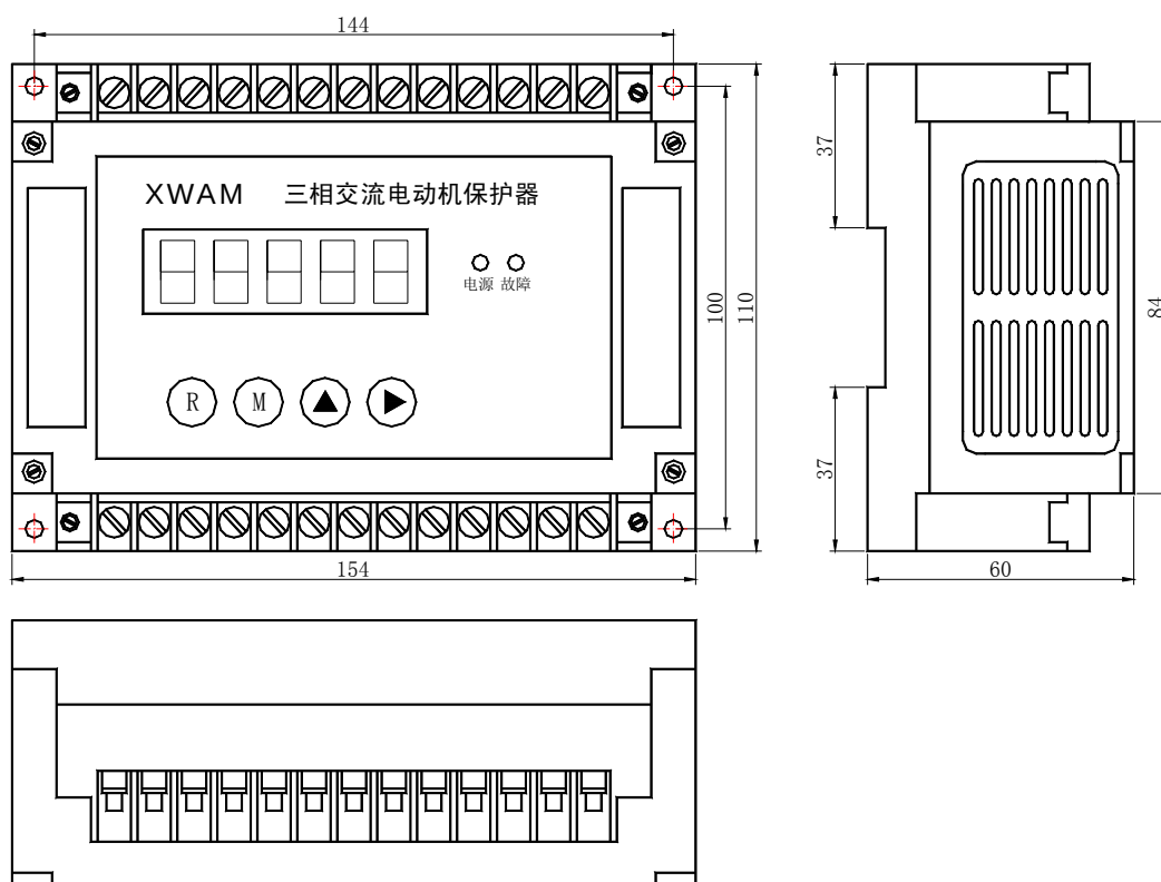
AMDGH-□/D541 系列电动机保护器主单元外形及安装孔尺寸
