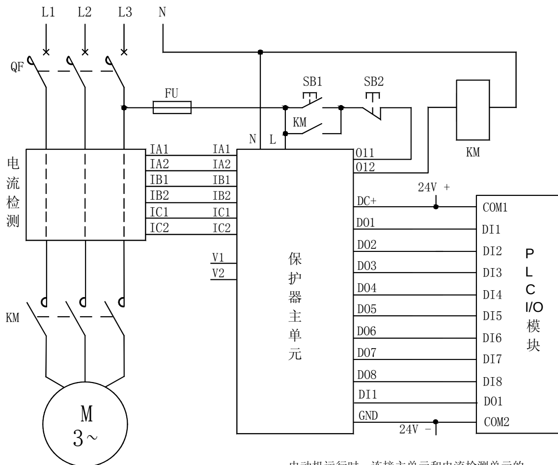
AMDGH-□/D541 系列电动机保护器 DO 连接 PLC 电气原理图
