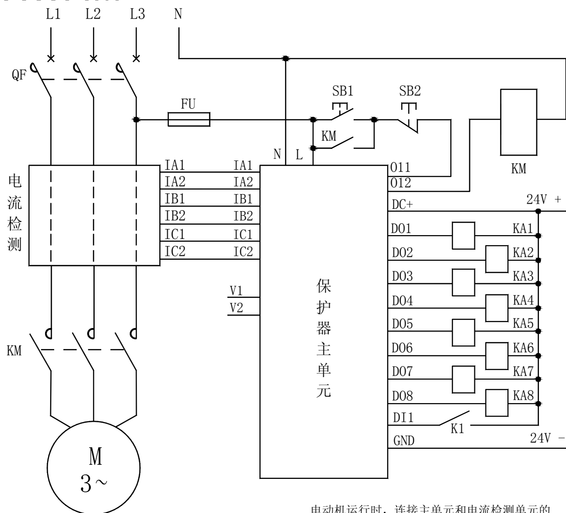
AMDGH-□/D541 系列电动机保护器 D0 连接继电器电气原理图
