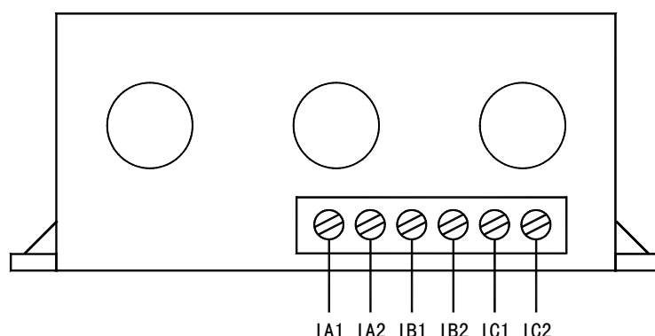
AMDGH-□/541 系列保护器电流检测单元接线端子图
