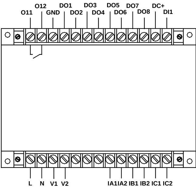
AMDGH-□/D541 系列保护器主单元接线端子图
