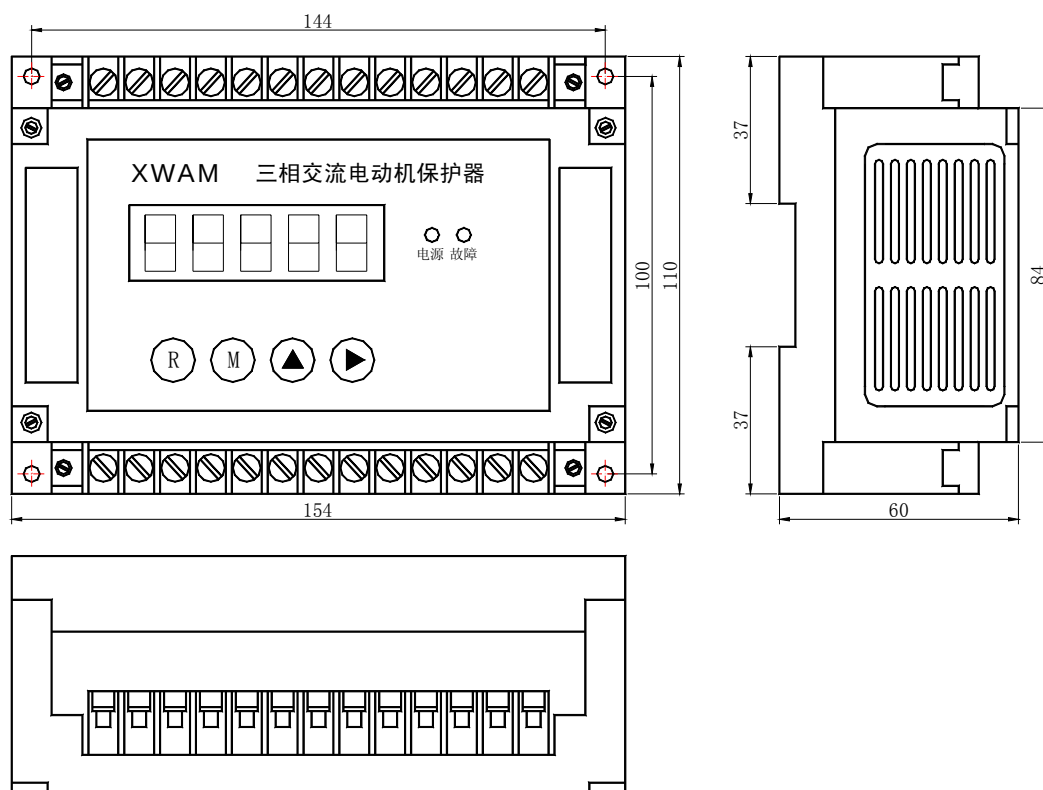
AMDGH-□/D601 系列电动机保护器主单元外形及安装孔尺寸
