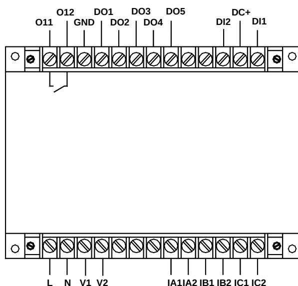
AMDGH-□/D601 系列保护器主单元接线端子图
