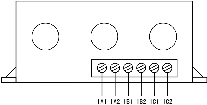
AMDGH-□/D601 系列保护器电流检测单元接线端子图
