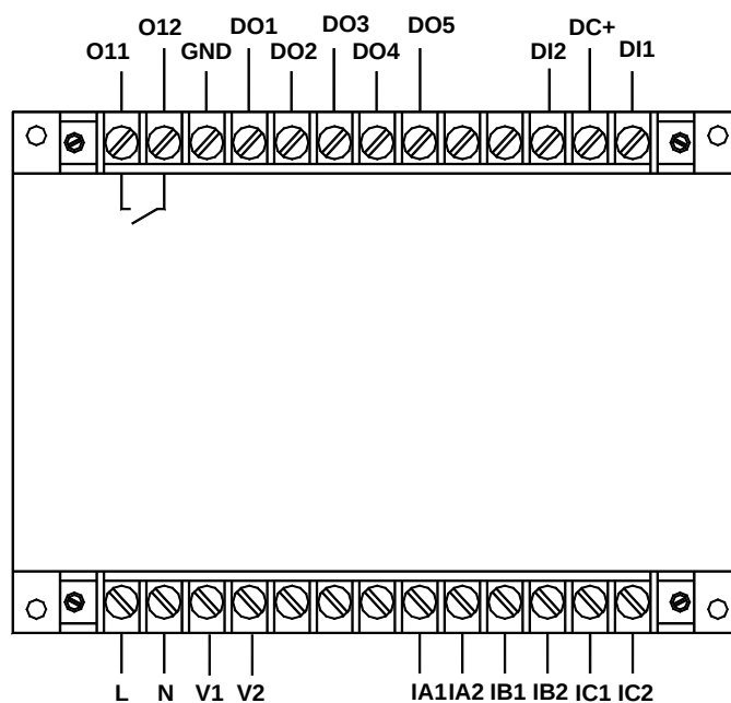
AMDGH-□/□/D621 系列保护器主单元接线端子图
