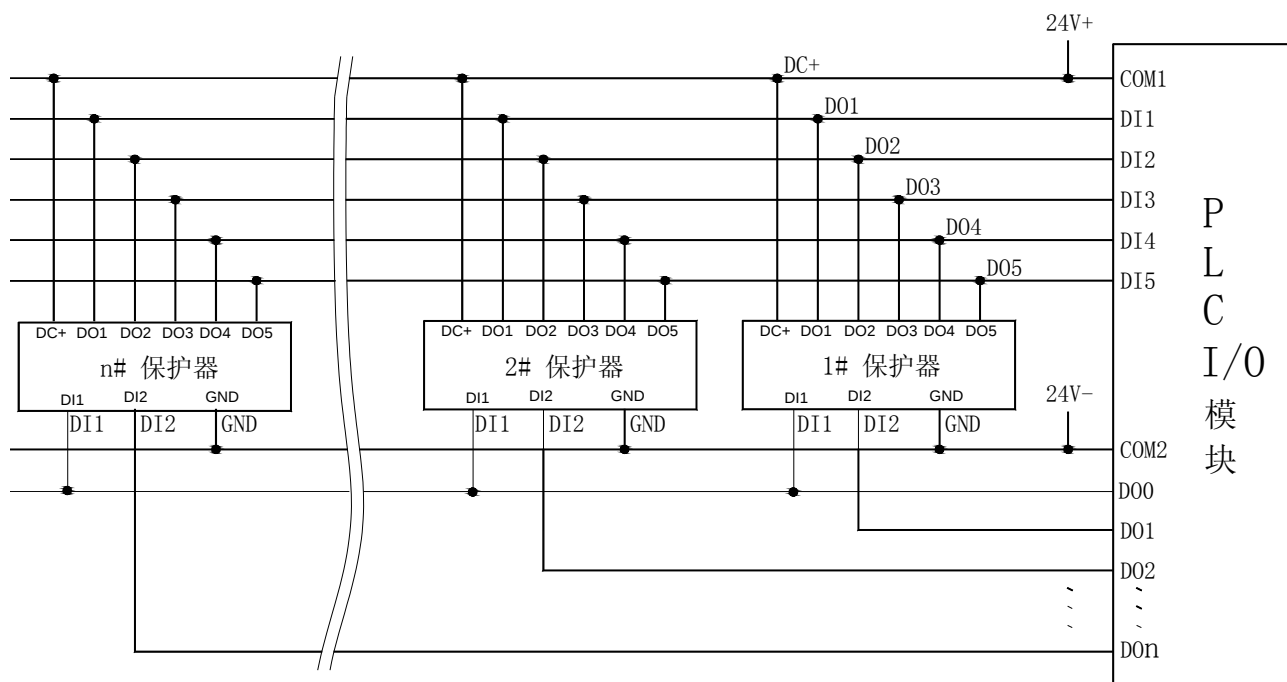
PLC 读取多台 AMDGH-□/D621 系列电动机保护器电气原理图
