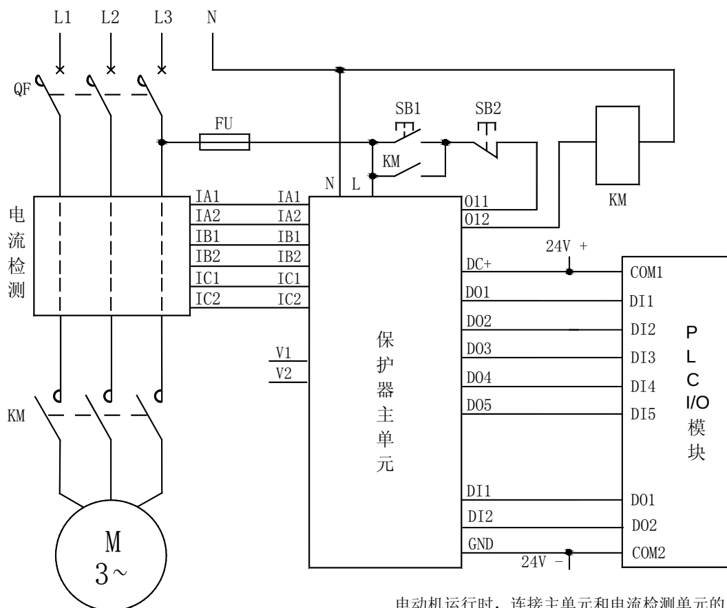
AMDGH-□/D621 系列电动机保护器 D0 连接 PLC 电气原理图
