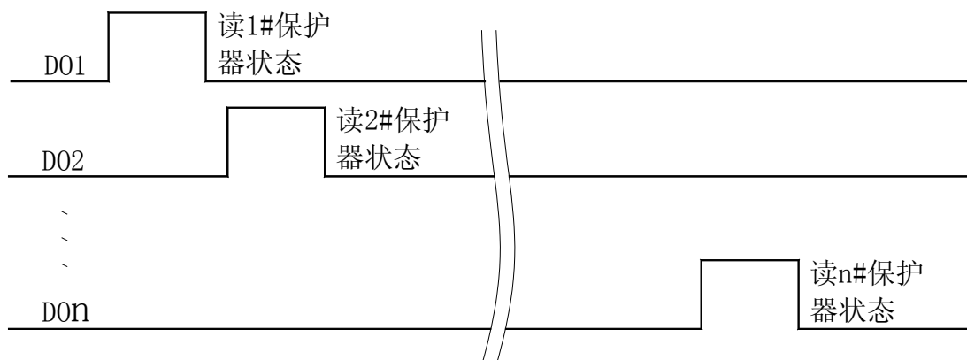
PLC 读取多台 AMDGH-□/D621 系列电动机保护器时序图
