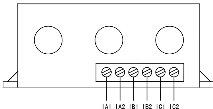
AMDGH-□/□/D621 系列保护器电流检测单元接线端子图
