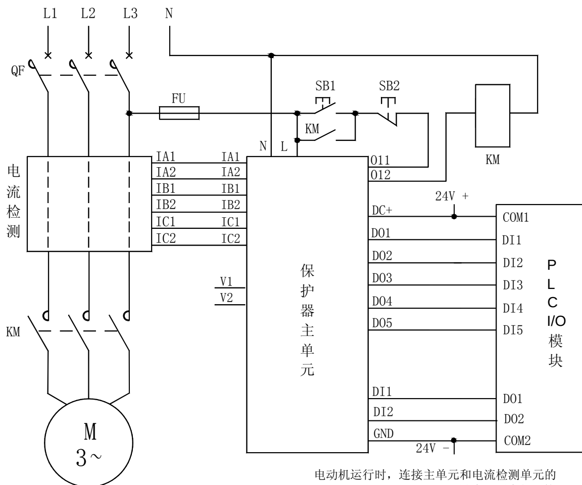
AMDGH-□/D631 系列电动机保护器 DO 连接 PLC 电气原理图
