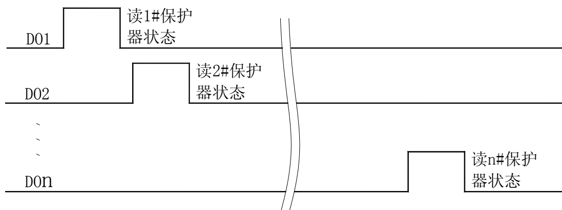
PLC 读取多台 AMDGH-□/D631 系列电动机保护器时序图
