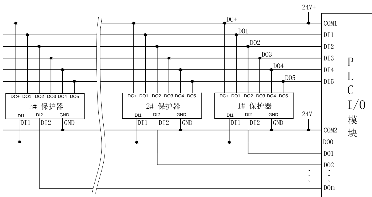
PLC 读取多台 AMDGH-□/D631 系列电动机保护器电气原理图
