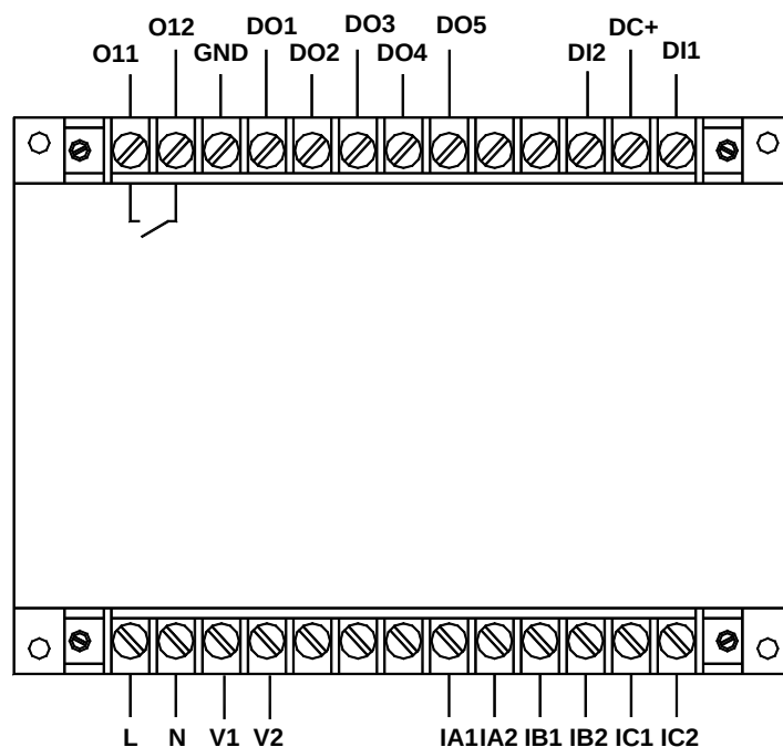
AMDGH-□/D631 系列保护器主单元接线端子图
