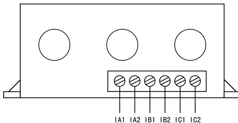
AMDGH-□/D631 系列保护器电流检测单元接线端子图
