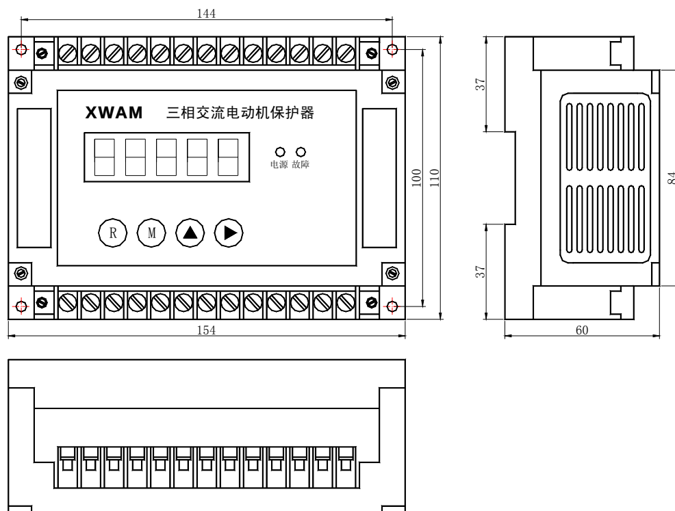
AMDGH-□/ D701 系列电动机保护器主单元外形及安装孔尺寸
