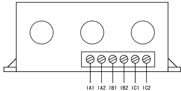
AMDGH-□/D741 系列保护器电流检测单元接线端子图
