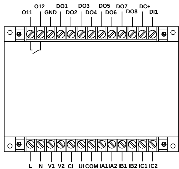
AMDGH-□/D741 系列保护器主单元接线端子图
