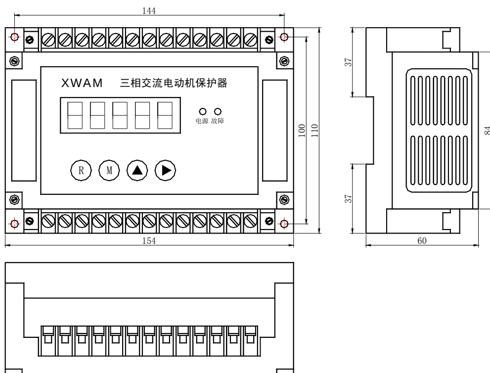
AMDGH-□/D741 系列电动机保护器主单元外形及安装孔尺寸
