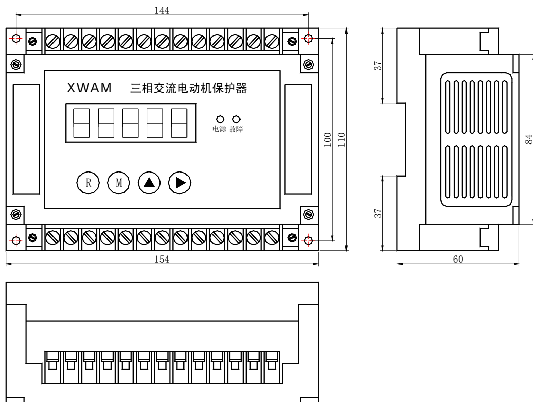
AMDGH-□/D821 系列电动机保护器主单元外形及安装孔尺寸
