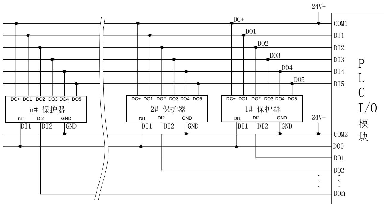
PLC 读取多台 AMDGH-□/D821 系列电动机保护器电气原理图
