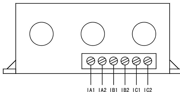
AMDGH-□/D821 系列保护器电流检测单元接线端子图
