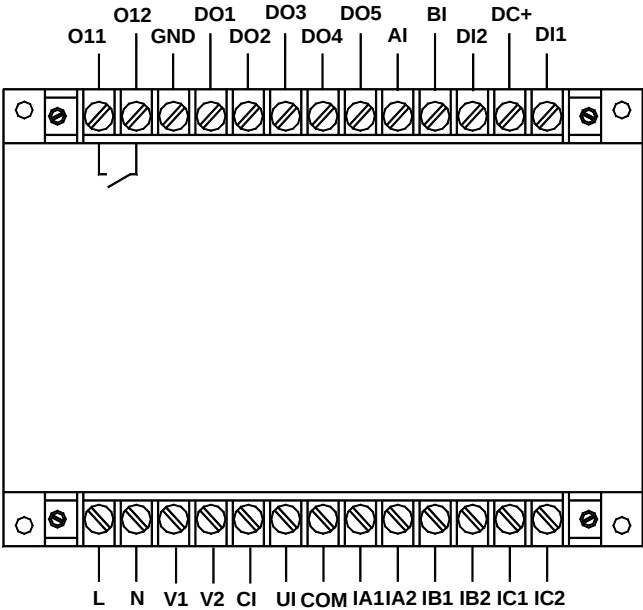
AMDGH-□/D821 系列保护器主单元接线端子图
