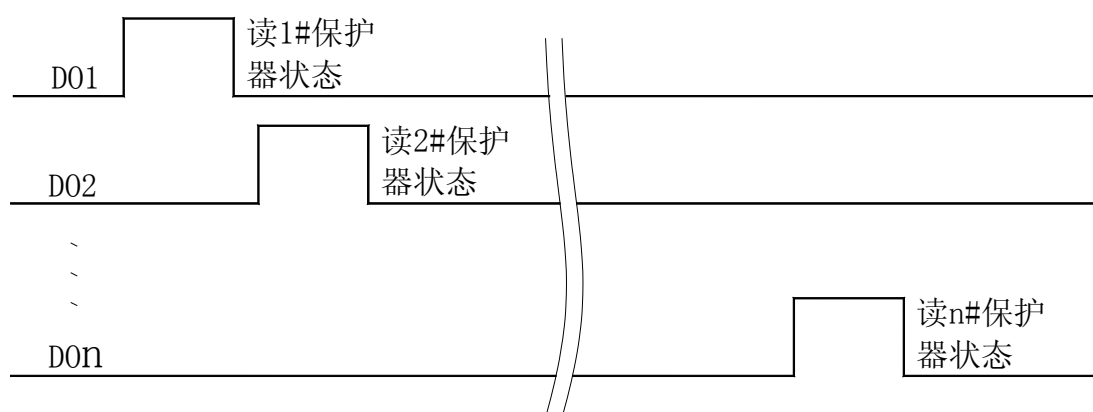
PLC 读取多台 AMDGH-□/D821 系列电动机保护器时序图
