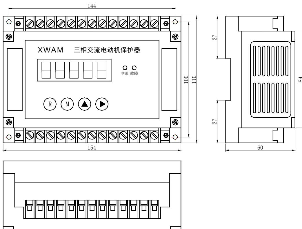
AMDGH-□/D831 系列电动机保护器主单元外形及安装孔尺寸
