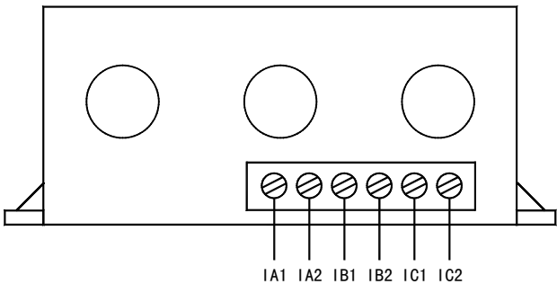
AMDG-□/D831 系列保护器电流检测单元接线端子图
