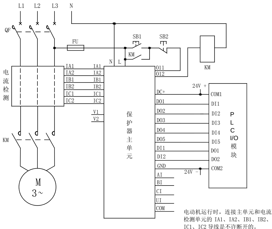
AMDGH-□/D841 系列电动机保护器 DO 连接 PLC 电气原理图
