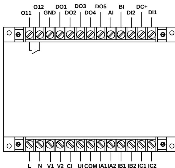
AMDG-□/□D841 系列保护器主单元接线端子图
