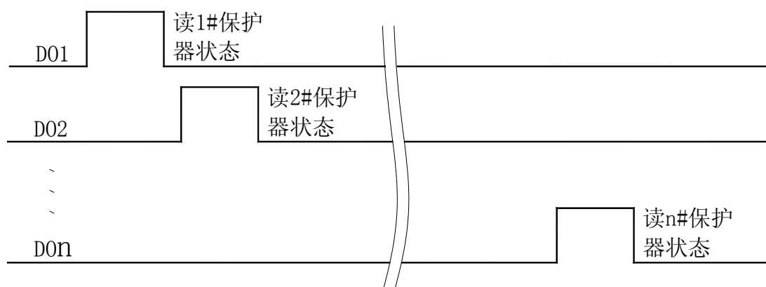
PLC 读取多台 AMDGH-□/D841 系列电动机保护器时序图
