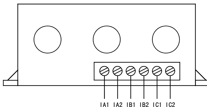
AMDG-□/□D841 系列保护器电流检测单元接线端子图
