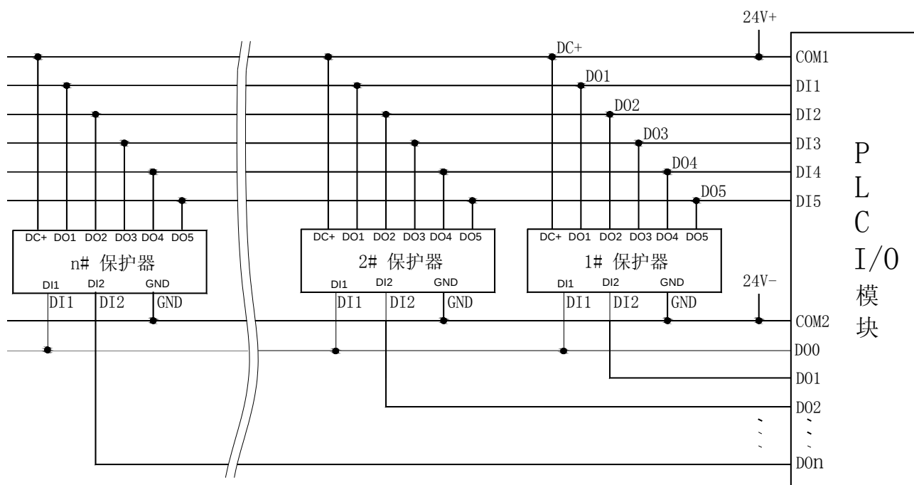
PLC 读取多台 AMDGH-□/D841 系列电动机保护器电气原理图
