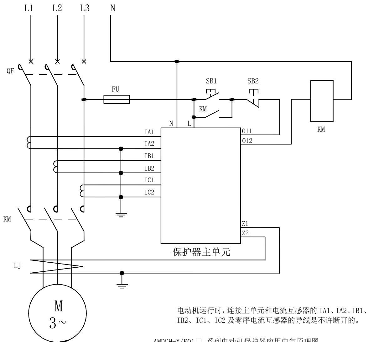
AMDGH-X/E01□ 系列电动机保护器应用电气原理图
