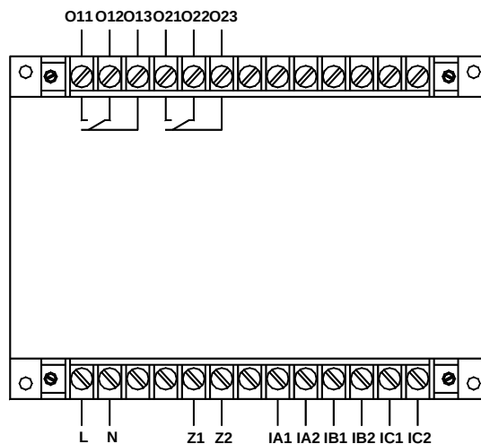
AMDGH-X/E012 系列保护器主单元接线端子图
