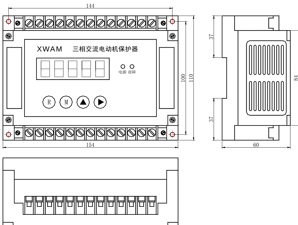
AMDGHH-X/E01□ 系列电动机保护器主单元外形及安装孔尺寸
