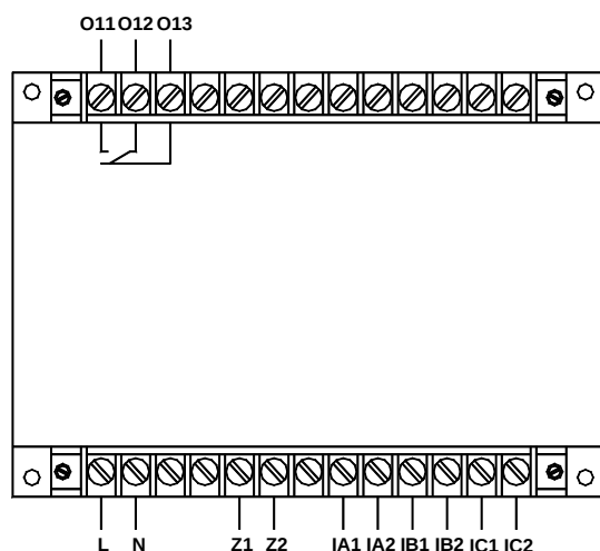
AMDGH-X/E011 系列保护器主单元接线端子图
