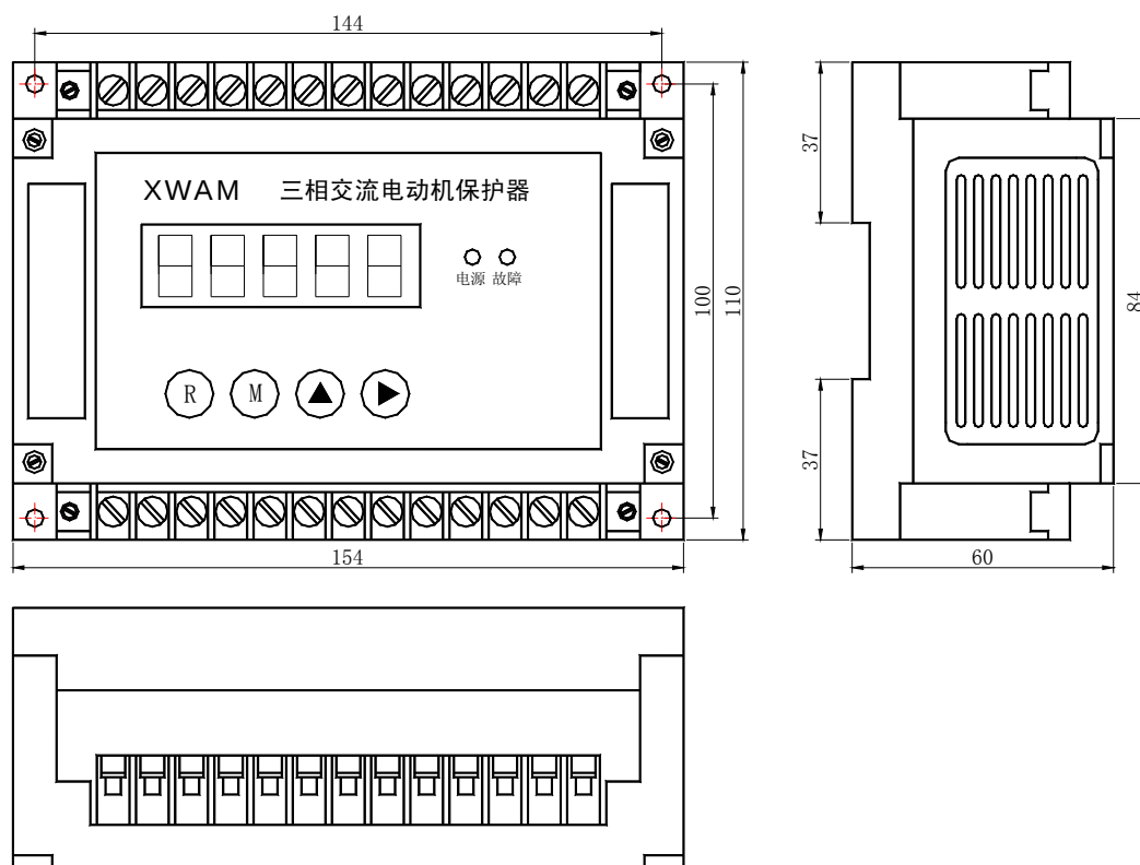
AMDGH-X/E701 系列电动机保护器主单元外形及安装孔尺寸
