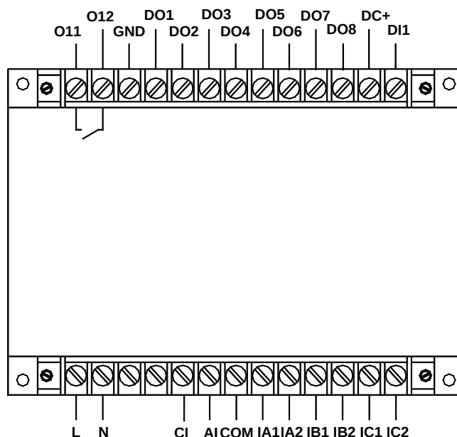
AMDGH-X/E701 系列保护器主单元接线端子图
