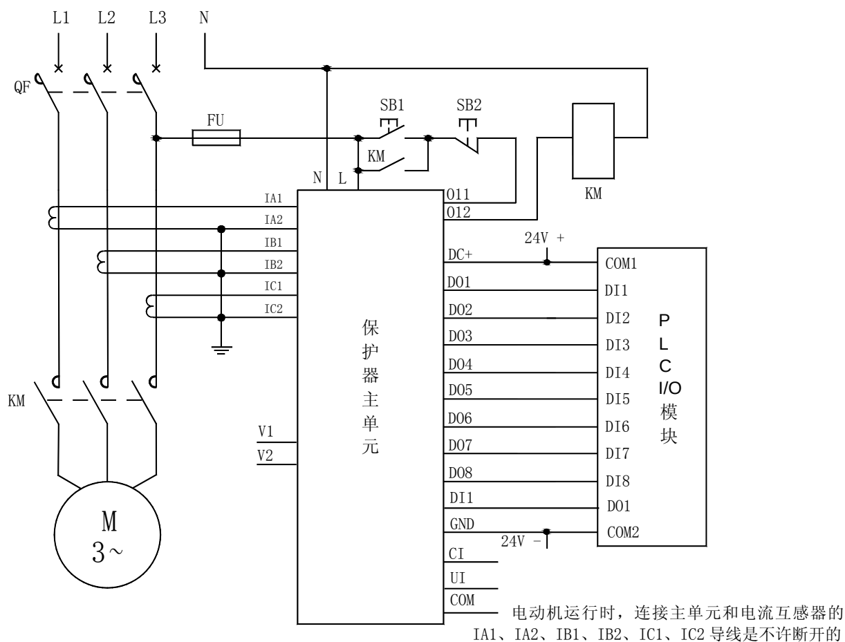
AMDGH-X/F721 系列电动机保护器 D0 连接 PLC 电气原理图
