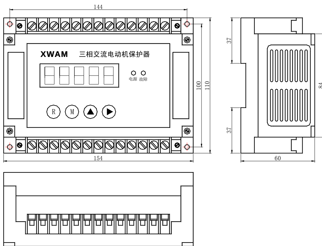
AMDGH-X/F721 系列电动机保护器主单元外形及安装孔尺寸
