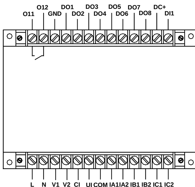
AMDGH-X/F721 系列保护器主单元接线端子图
