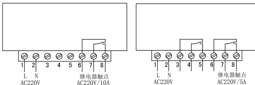
AMDL-□/0041 系列 100A 及小于 100A 接线端子图
