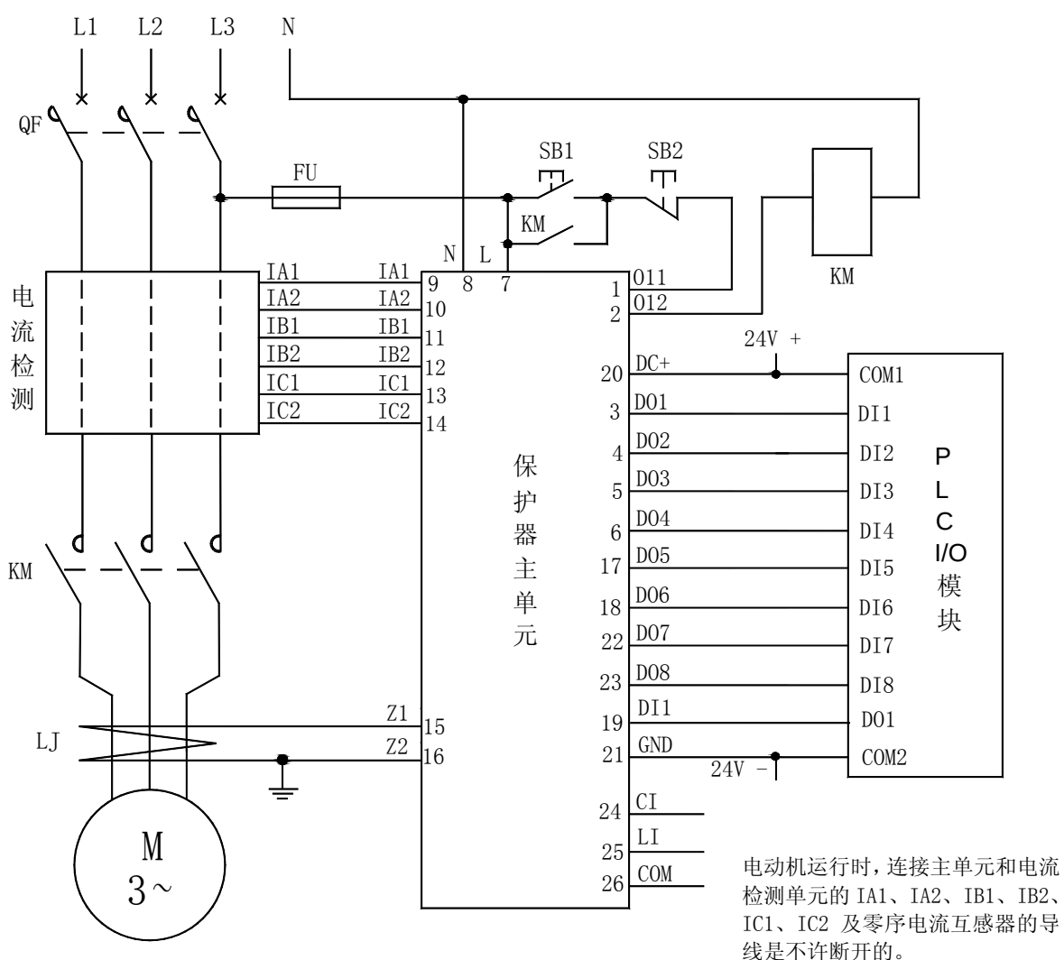
AMDP-□/C751 系列电动机保护器 D0 连接 PLC 电气原理图
