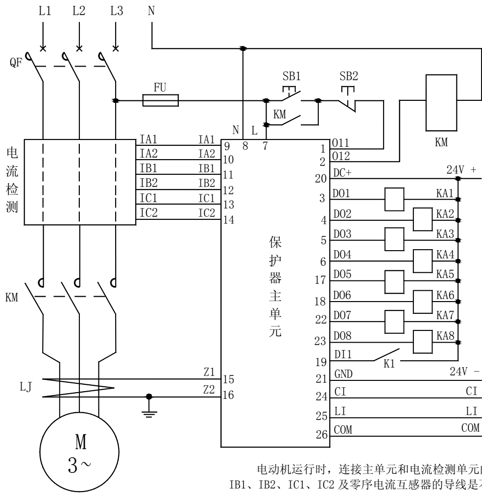
AMDP-□/751 系列电动机保护器 D0 连接继电器电气原理图
