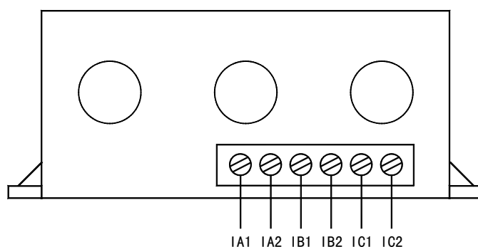
AMDP-□/751 系列保护器电流检测单元接线端子图
