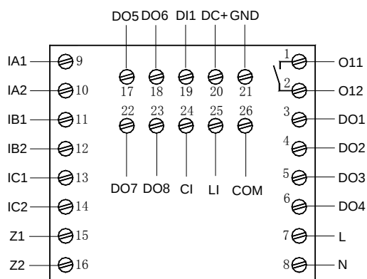
AMDP-□/751 系列保护器主单元接线端子图
