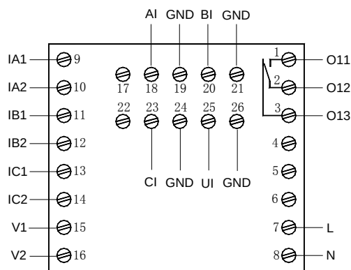
AMDP-□/D141 系列保护器主单元接线端子图
