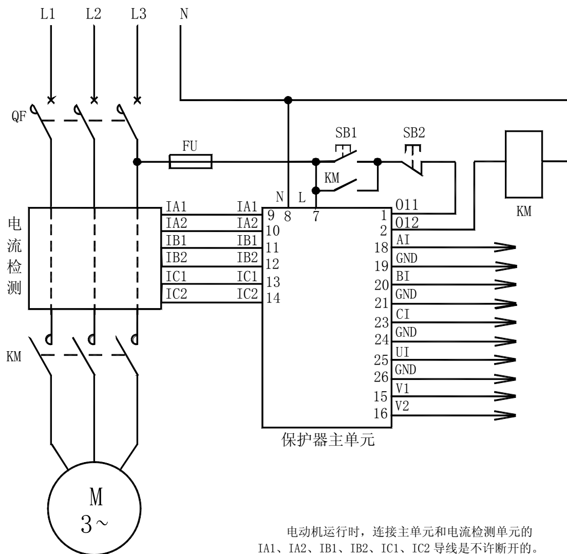
AMDP-□/D14□ 系列电动机保护器应用电气原理图
