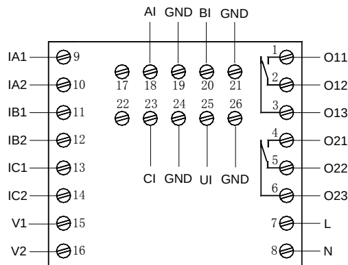
AMDP-□/D142 系列保护器主单元接线端子图
