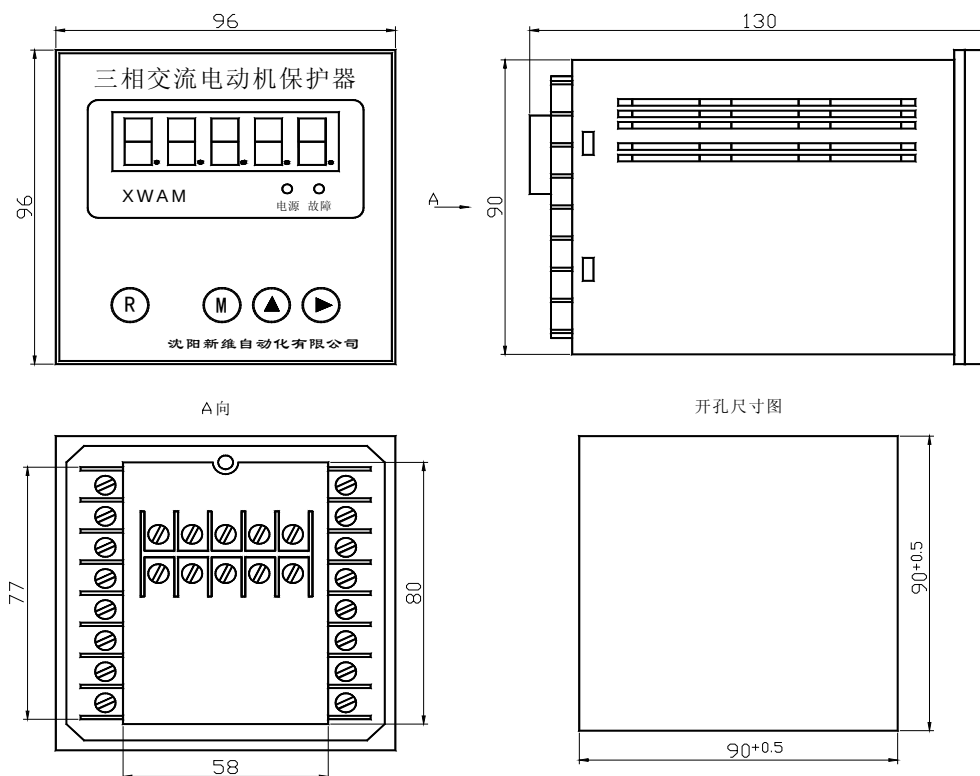
AMDP-□/D14□ 系列电动机保护器主单元外形及安装孔尺寸
