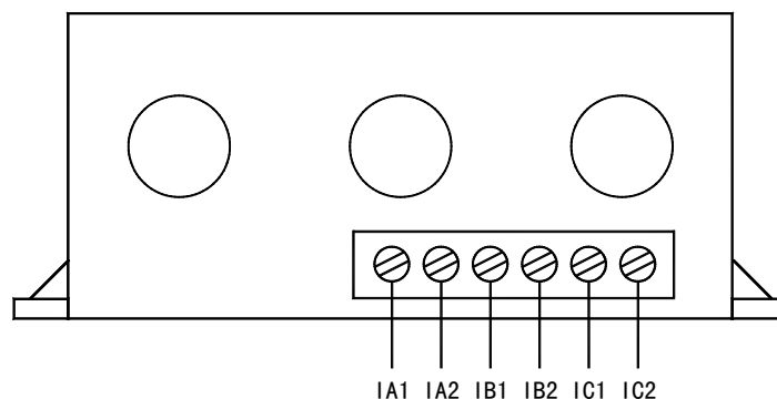
AMDP-□/D14□ 系列保护器电流检测单元接线端子图
