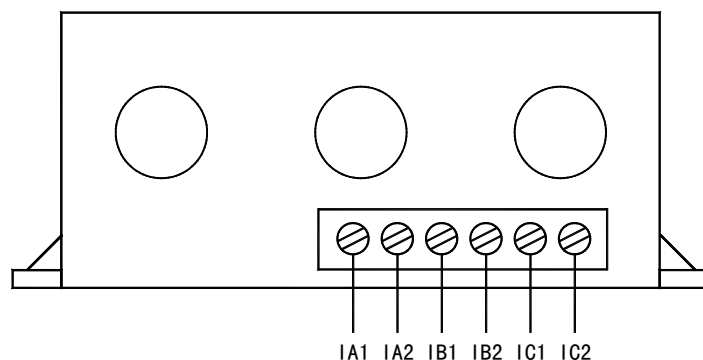
AMDP-□/D20□ 系列保护器电流检测单元接线端子图
