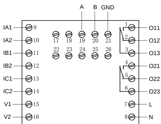
AMDP-□/D202 系列保护器主单元接线端子图
