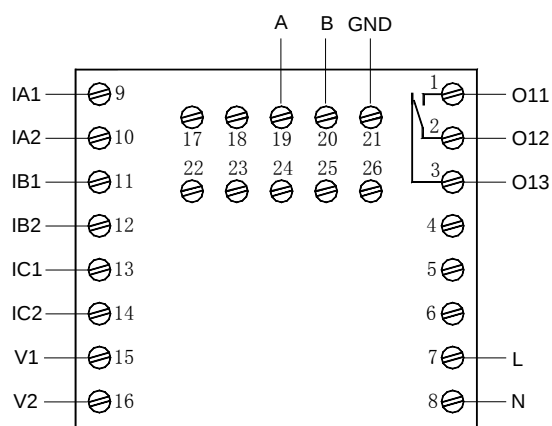
AMDP-□/D201 系列保护器主单元接线端子图
