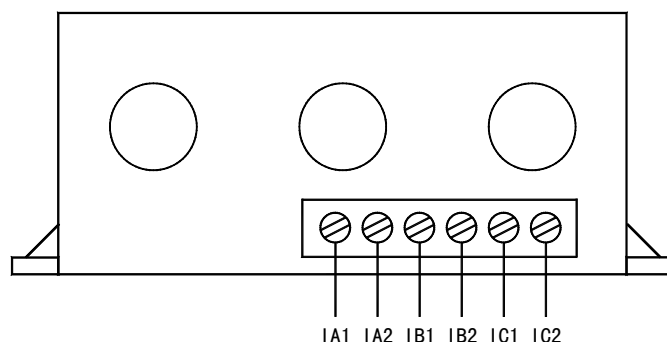
AMDP-□/D23□ 系列保护器电流检测单元接线端子图
