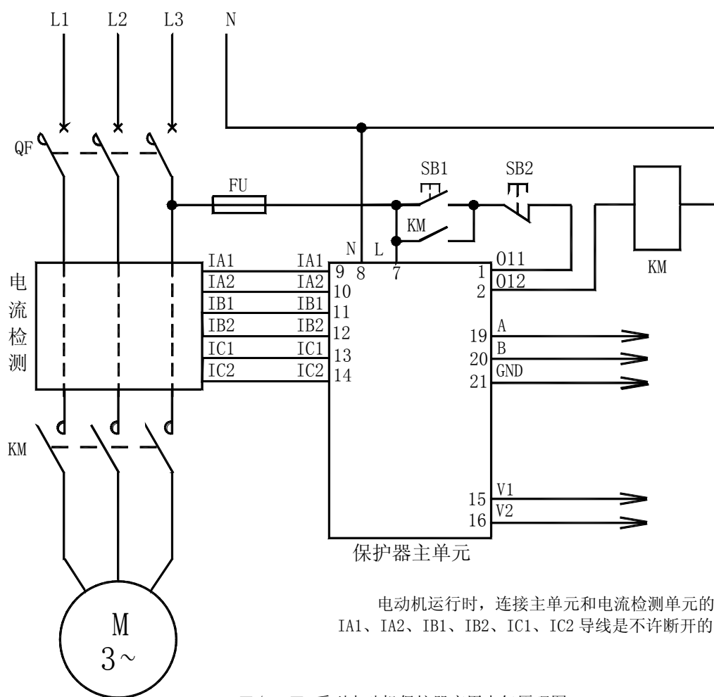
AMDP-□/ D23□ 系列电动机保护器应用电气原理图
