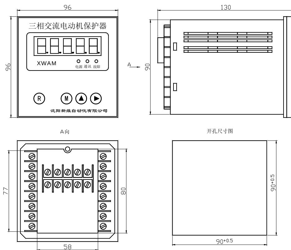
AMDP-□/D23□ 系列电动机保护器主单元外形及安装孔尺寸
