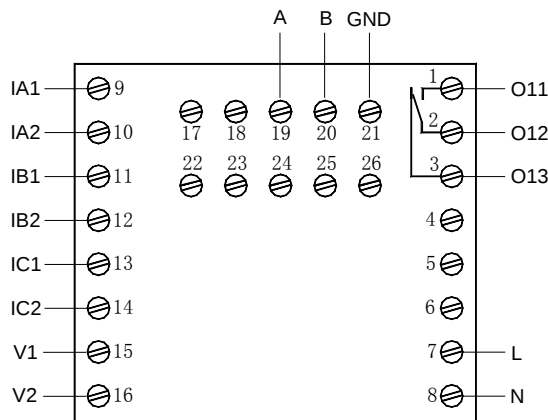
AMDP-□/D231 系列保护器主单元接线端子图
