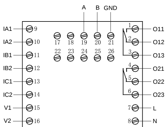
AMDP-□/D232 系列保护器主单元接线端子图
