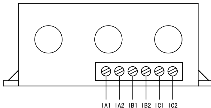
AMDP-□/D25□ 系列保护器电流检测单元接线端子图
