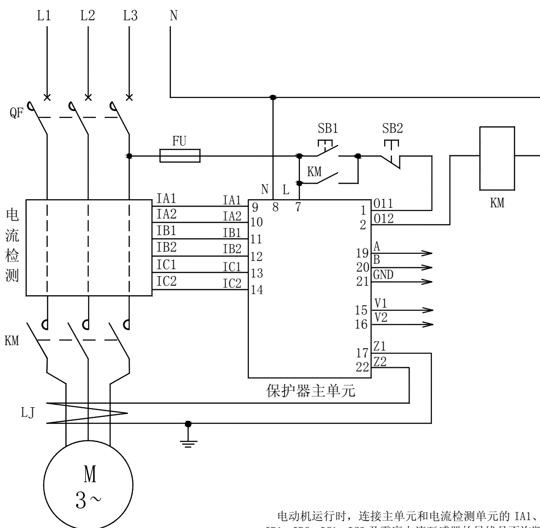
AMDP-□/D25□ 系列电动机保护器应用电气原理图
