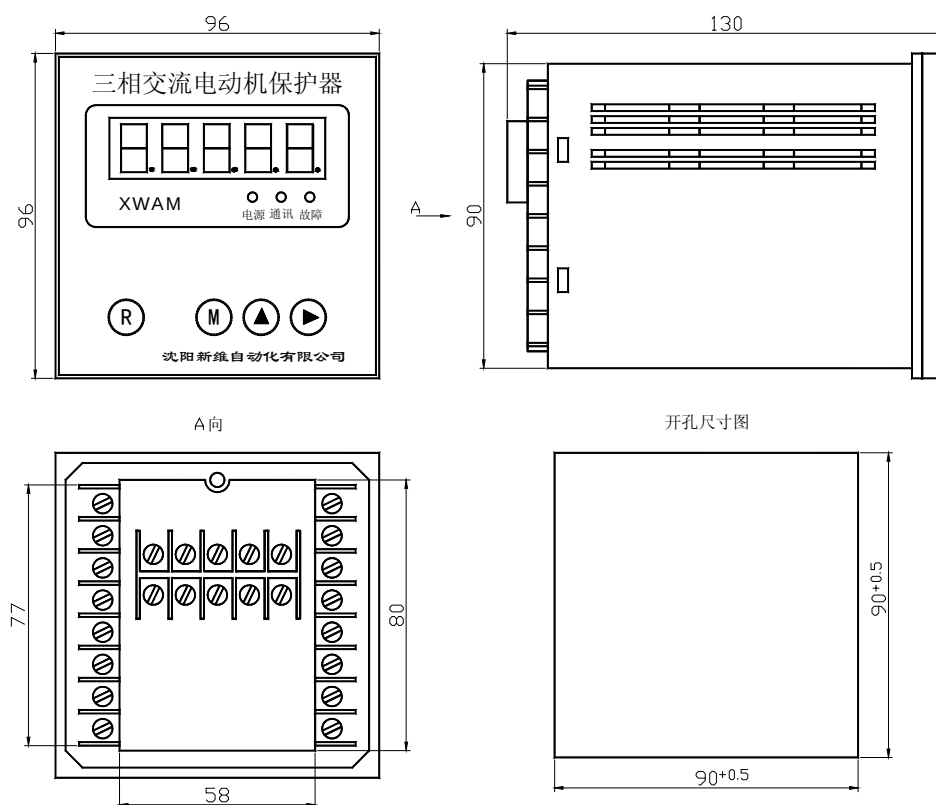
AMDP-□/D25□ 系列电动机保护器主单元外形及安装孔尺寸
