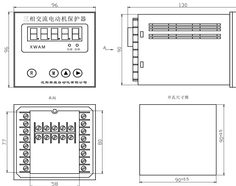
AMDP-□/501 系列电动机保护器主单元外形及安装孔尺寸
