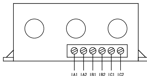
AMDP-□/501 系列保护器电流检测单元接线端子图
