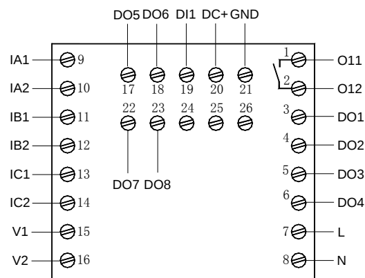
AMDP-□/D501 系列保护器主单元接线端子图
