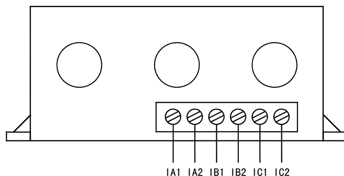
AMDP-□/DO21 系列保护器电流检测单元接线端子图
