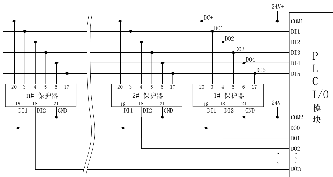
PLC 读取多台 AMDP-□/D621 系列电动机保护器电气原理图
