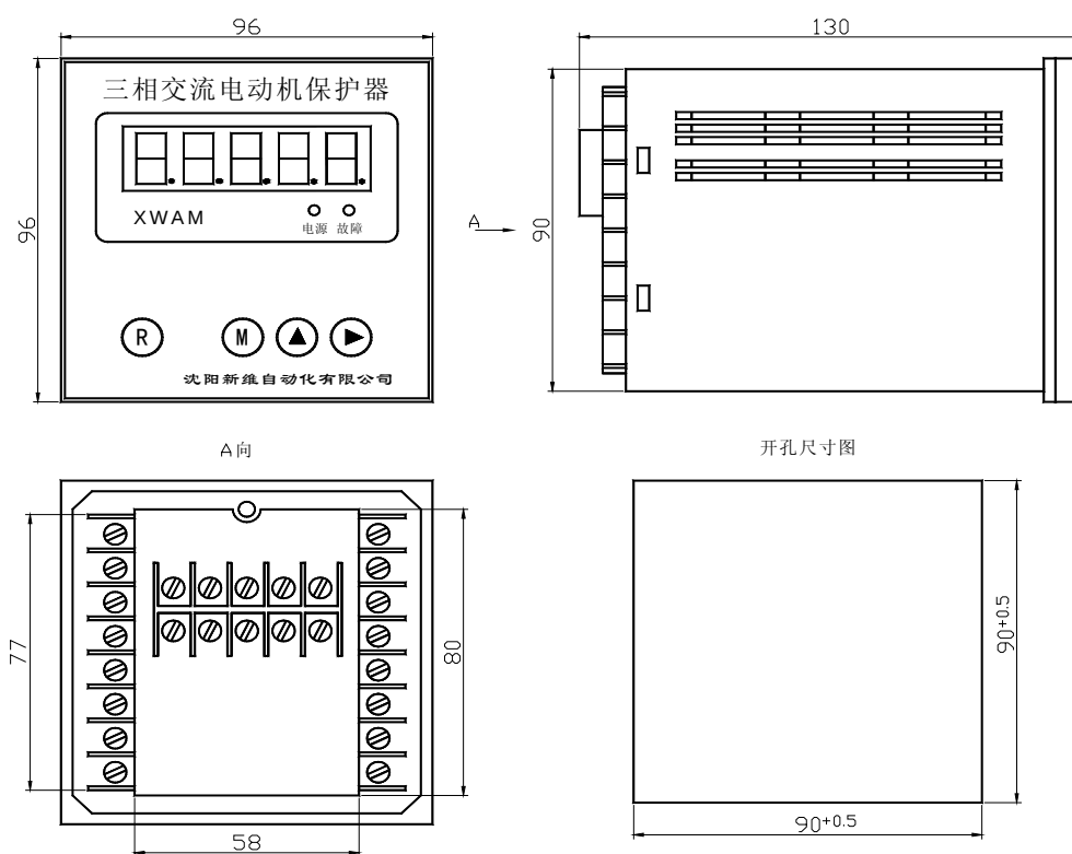
AMDP-□/D621 系列电动机保护器主单元外形及安装孔尺寸
