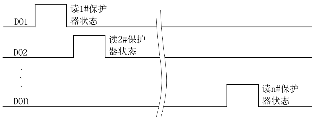
PLC 读取多台 AMDP-□/D621 系列电动机保护器时序图
