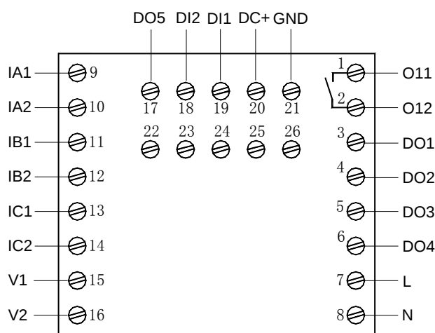
AMDP-□/DO21 系列保护器电流检测单元接线端子图
