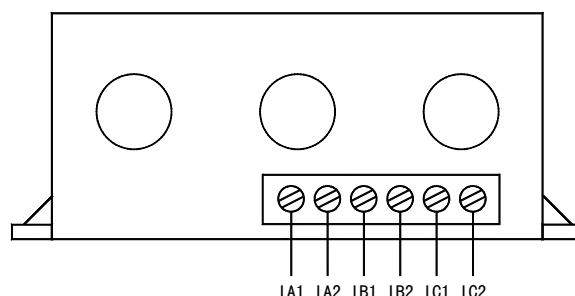
AMDP-□/731 系列保护器电流检测单元接线端子图
