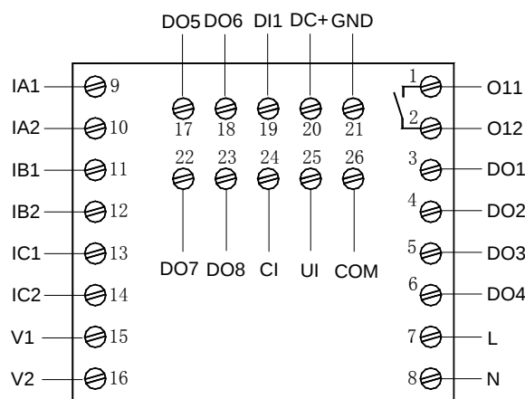
AMDP-□/731 系列保护器主单元接线端子图
