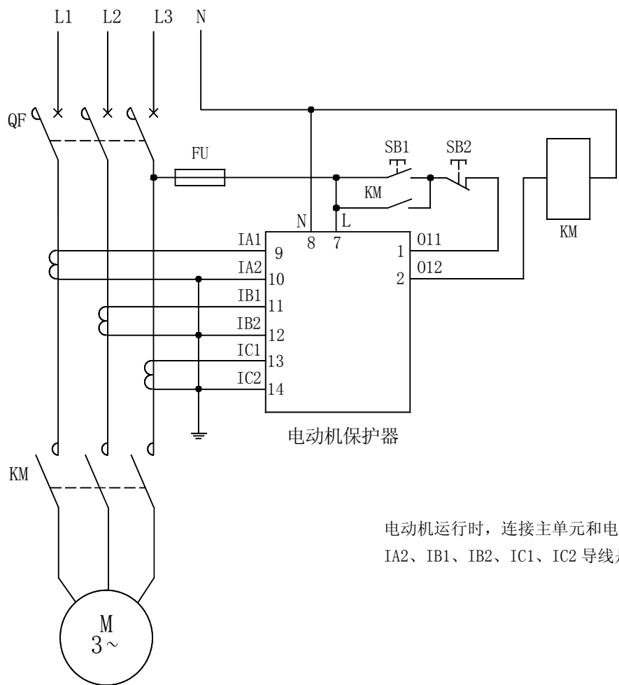
AMDP-X/E00□ 系列电动机保护器应用电气原理图
