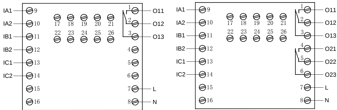
AMDP-X/E001 系列保护器主单元接线端子图
