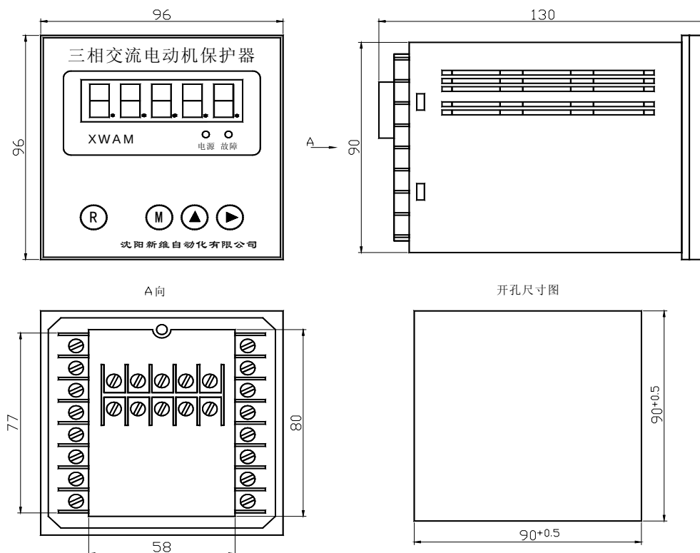
AMDP-X/E01□ 系列电动机保护器主单元外形及安装孔尺寸
