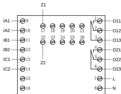
AMDP-X/E012 系列保护器主单元接线端子图
