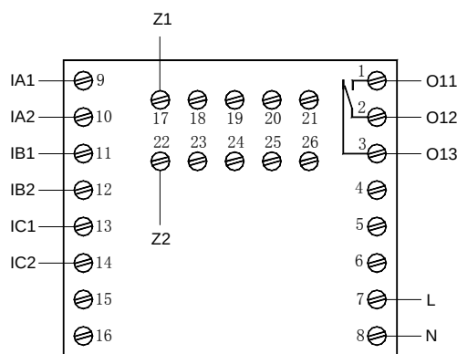
AMDP-X/E011 系列保护器主单元接线端子图
