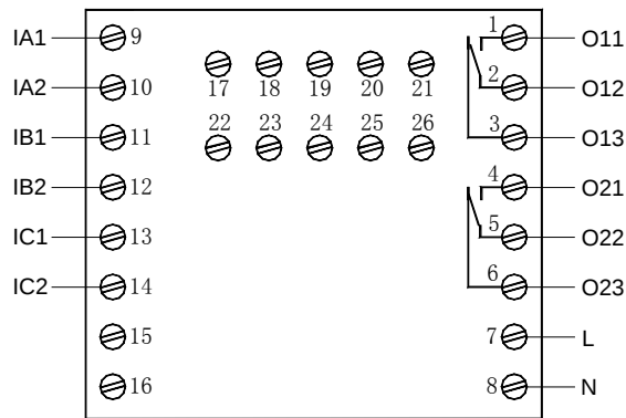
AMDP-X/E022 系列保护器主单元接线端子图
