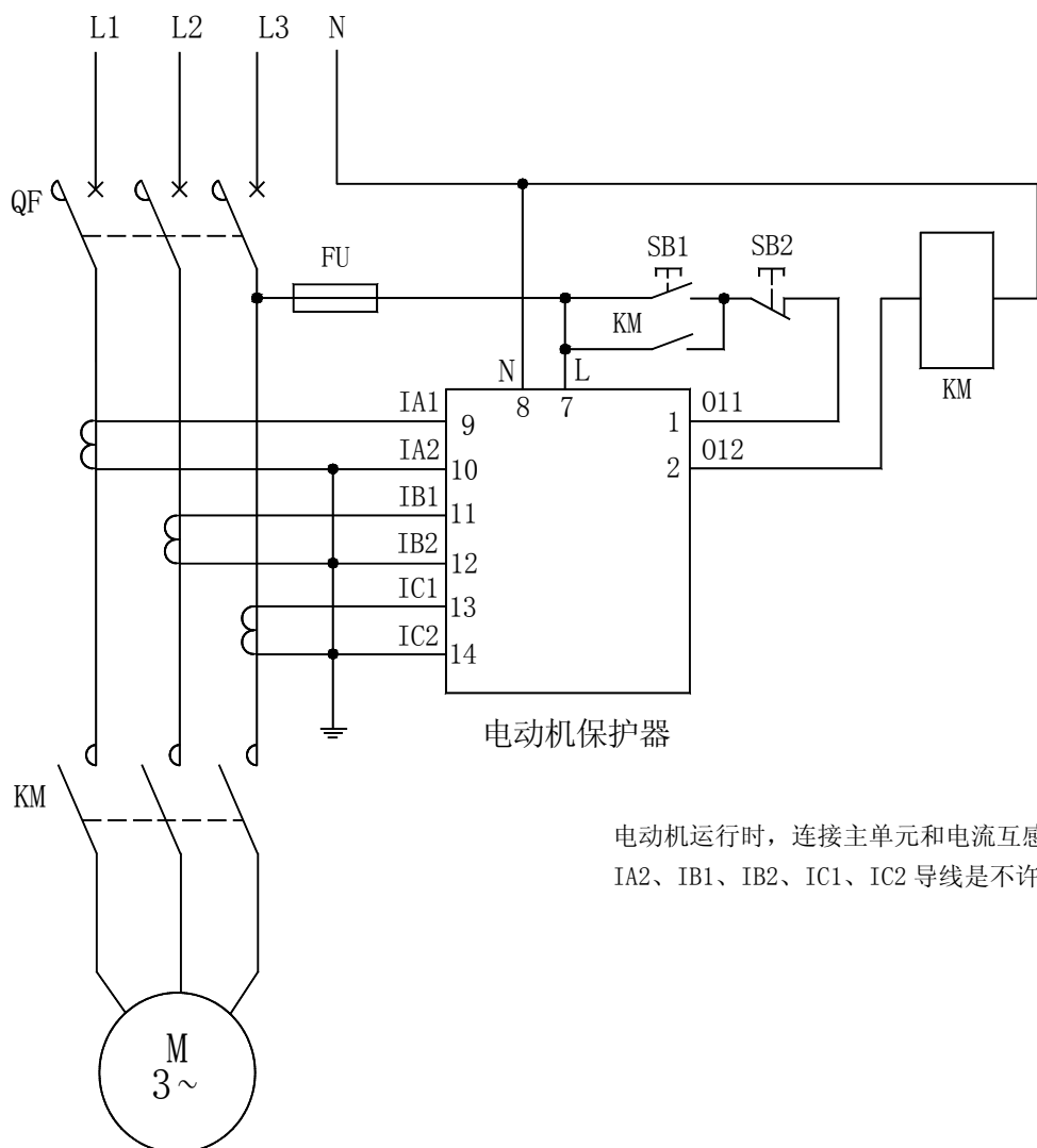
AMDP-X/E02□ 系列电动机保护器应用电气原理图
