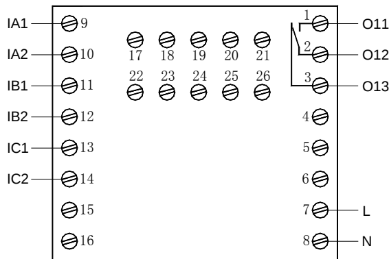
AMDP-X/E021 系列保护器主单元接线端子图
