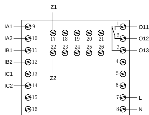
AMDP-X/E051 系列保护器主单元接线端子图
