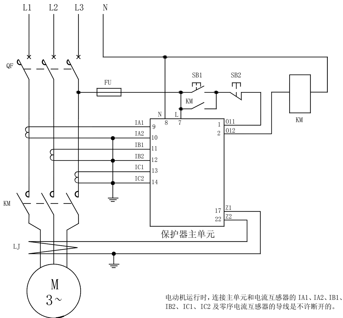
AMDP-X/E05□ 系列电动机保护器应用电气原理图
