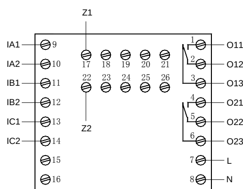
AMDP-X/E052 系列保护器主单元接线端子图
