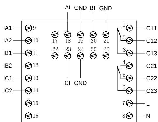
AMDP-X/E102 系列保护器主单元接线端子图
