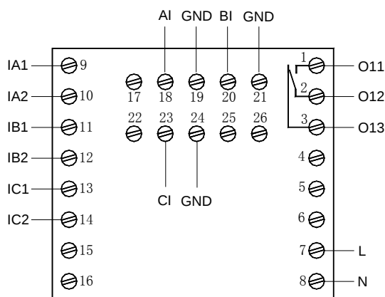
AMDP-X/E101 系列保护器主单元接线端子图
