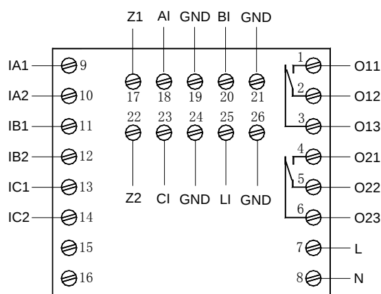
AMDP-X/E112 系列保护器主单元接线端子图
