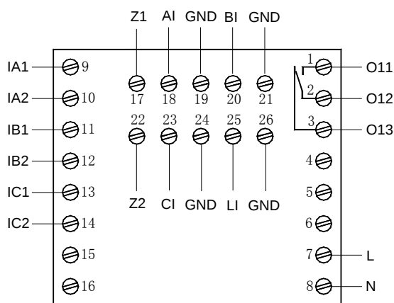
AMDP-X/E111 系列保护器主单元接线端子图
