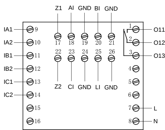
AMDP-X/E151 系列保护器主单元接线端子图
