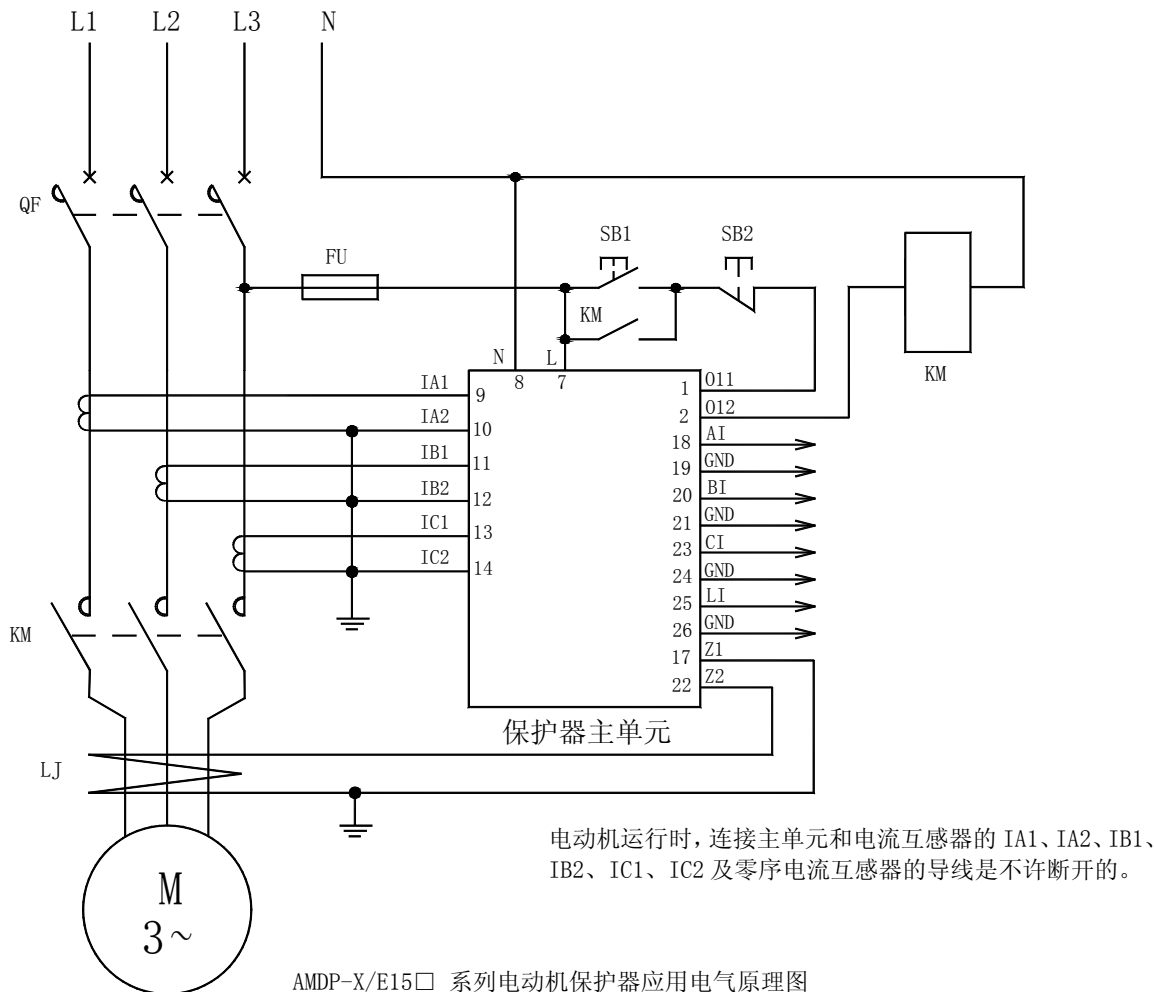
AMDP-X/E15□ 系列电动机保护器应用电气原理图
