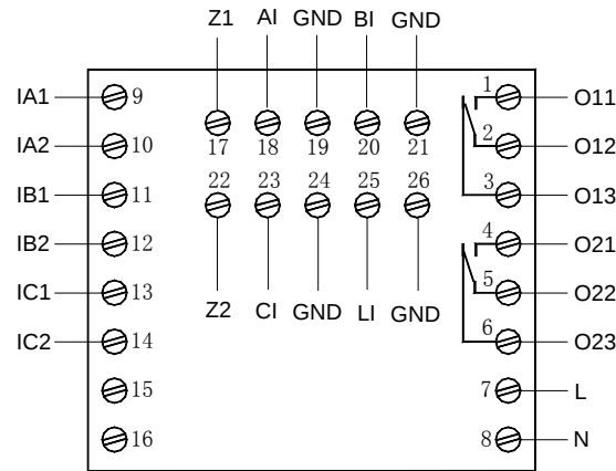
AMDP-X/E152 系列保护器主单元接线端子图
