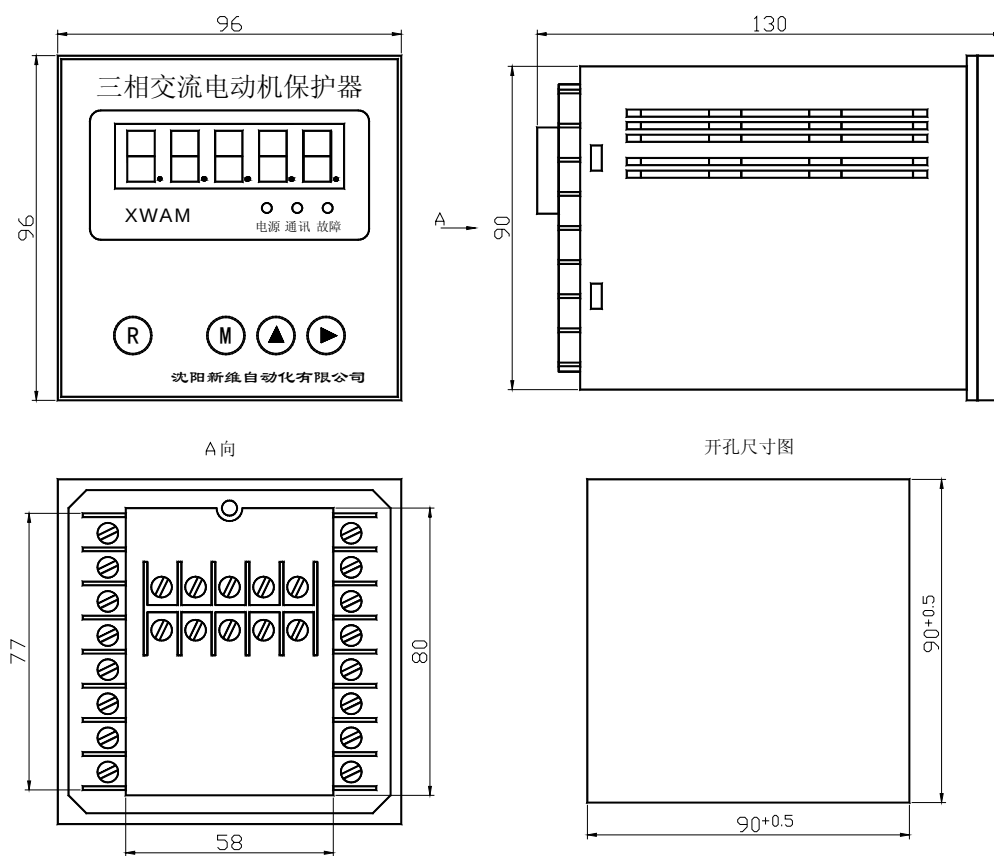
AMDP-X/E20□ 系列电动机保护器主单元外形及安装孔尺寸
