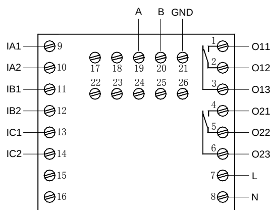
AMDP-X/E202 系列保护器主单元接线端子图
