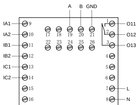
AMDP-X/E201 系列保护器主单元接线端子图
